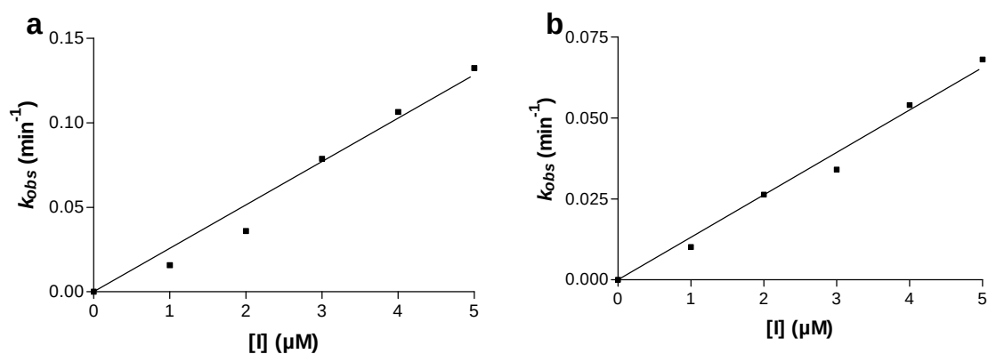
Figure 54: Inactivation du FXa par le LP 53 (1-5 \mu\text{M} ) : k_{obs}/[I] = 428 \pm 19.3 \text{ M}^{-1} \cdot \text{s}^{-1} ( a ) et par le LP 74 (1-5 \mu\text{M} ) : k_{obs}/[I] = 218.5 \pm 6.77 \text{ M}^{-1} \cdot \text{s}^{-1} ( b )
