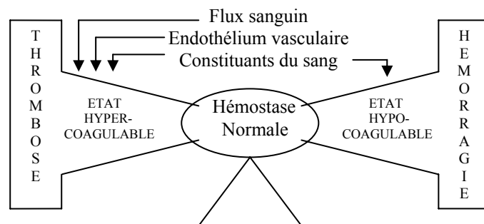
Figure 2 : Balance hémostatique
