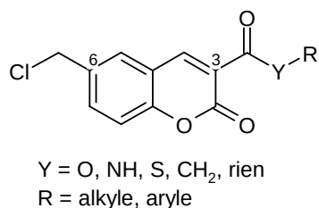
Figure 34 : Coumarines 3,6-disubstituées
