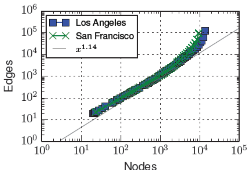
FIGURE 1 – Nombre d’arêtes en fonction du nombre de noeuds de Los Angeles et de San Francisco via les données des utilisateurs de l’application Foursquare. Source : [21]
