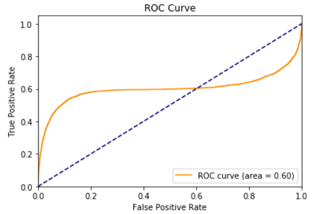
FIGURE 71 – Courbe ROC de Tokyo pour 85 % des données avec l’algorithme utilisant le coefficient de Jaccard pour la prédiction des arêtes
