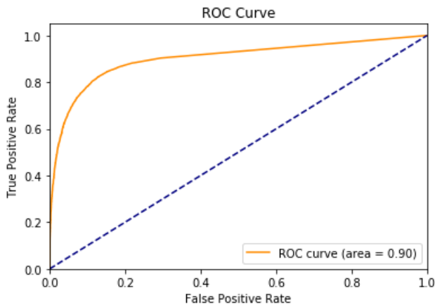
FIGURE 54 – Courbe ROC de New York pour 60 % des données avec l'algorithme utilisant le coefficient de Jaccard pour la prédiction des arêtes
