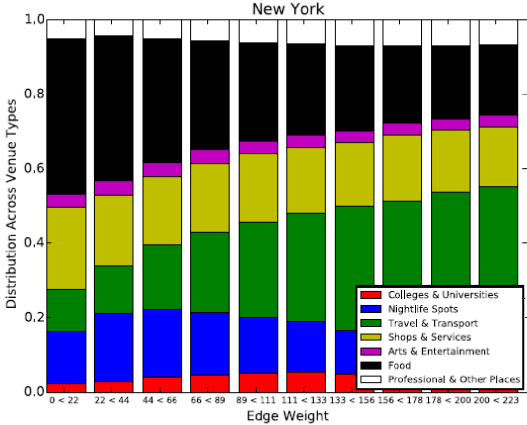
FIGURE 10 – Distribution par catégorie en fonction du poids des noeuds. Source : [21]
