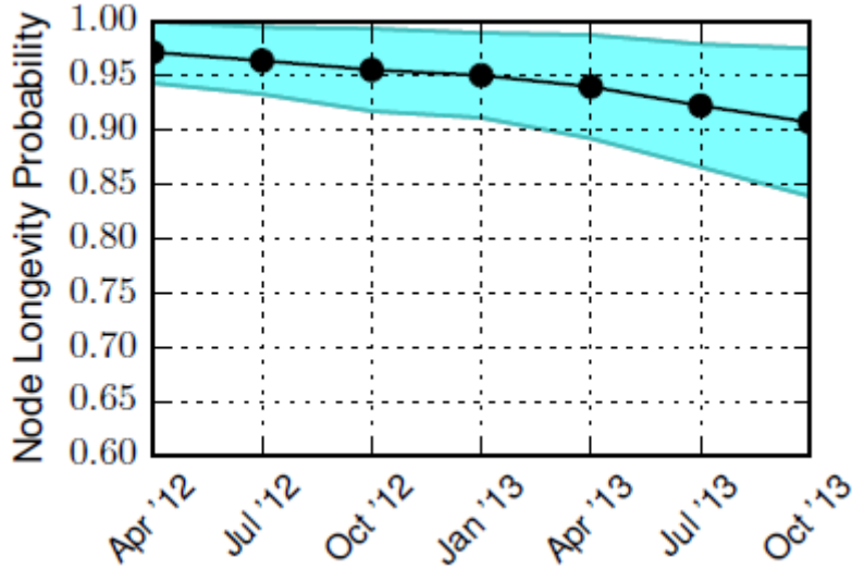
FIGURE 7 – Probabilité de persistance d'un noeud lors de la période de temps suivante. Source : [21]
