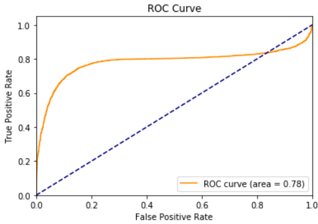
FIGURE 70 – Courbe ROC de New York pour 85 % des données avec l’algorithme utilisant le coefficient de Jaccard pour la prédiction des arêtes
