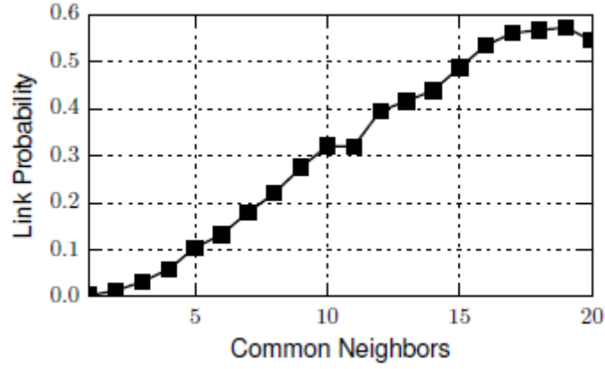
FIGURE 11 – Probabilité de la formation d’un lien dans la période de temps suivante en fonction du nombre de voisins partagés entre deux noeuds pour Chicago. Source : [21]
