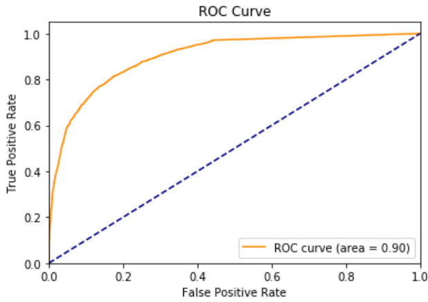
FIGURE 46 – Courbe ROC de New York pour 85 % des données avec l’algorithme utilisant le coefficient de Jaccard pour la prédiction des arêtes
