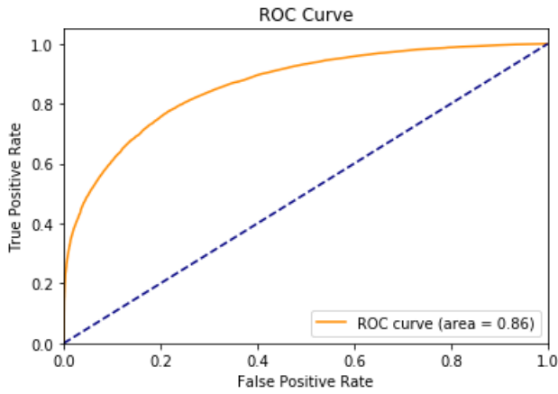
FIGURE 66 – Courbe ROC de New York pour 60 % des données avec l'algorithme utilisant le coefficient de Jaccard pour la prédiction des arêtes
