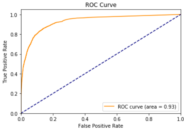
FIGURE 58 – Courbe ROC de New York pour 85 % des données avec l'algorithme utilisant le coefficient de Jaccard pour la prédiction des arêtes
