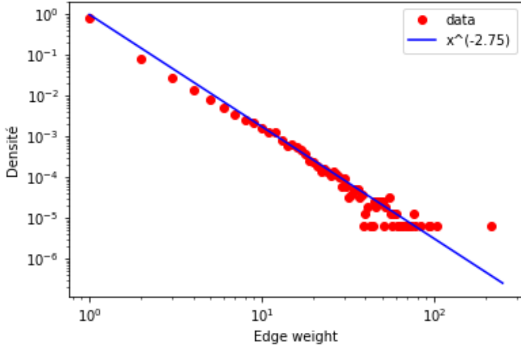
FIGURE 26 – Répartition des arêtes en fonction de leur poids pour la ville de New York.
