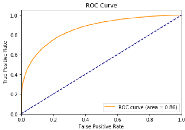
FIGURE 68 – Courbe ROC de New York pour 35 % des données avec l'algorithme utilisant le coefficient de Jaccard pour la prédiction des arêtes
