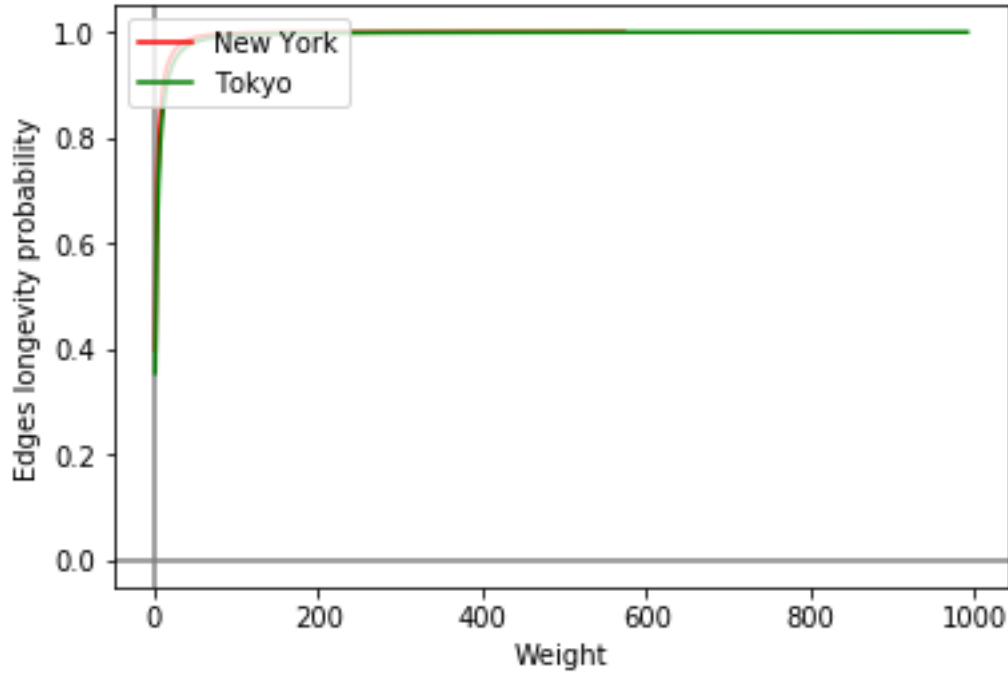
FIGURE 43 – Persistance des arêtes en fonction du poids de celles-ci entre deux périodes de temps successives
