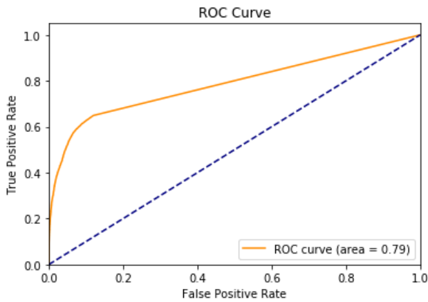
FIGURE 62 – Courbe ROC de New York pour 35 % des données avec l’algorithme utilisant le coefficient de Jaccard pour la prédiction des arêtes
