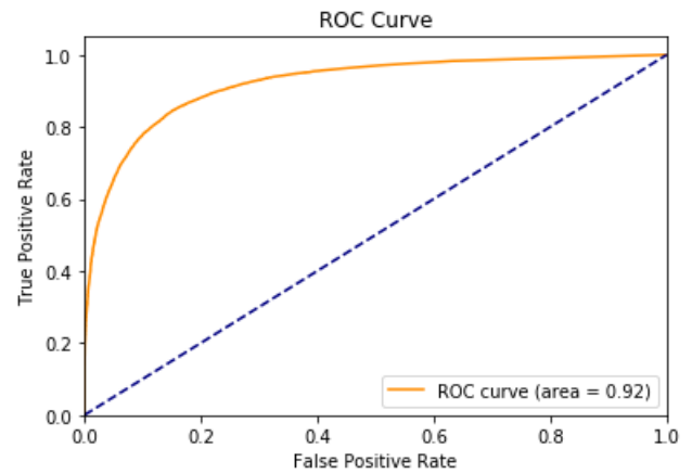
FIGURE 55 – Courbe ROC de Tokyo pour 60 % des données avec l'algorithme utilisant le coefficient de Jaccard pour la prédiction des arêtes
