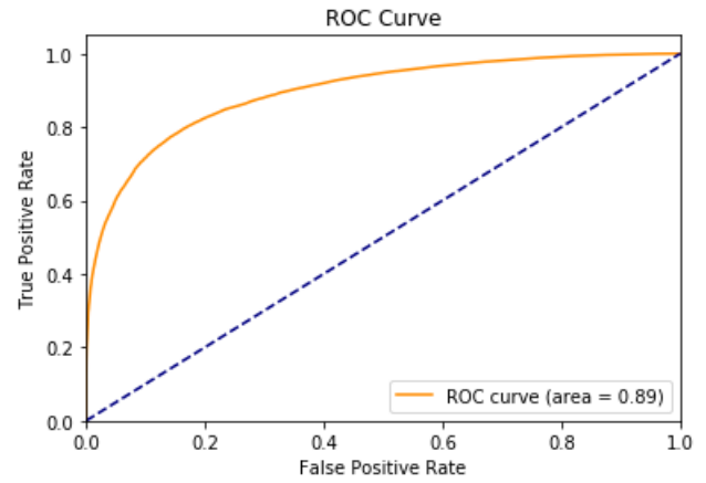
FIGURE 67 – Courbe ROC de Tokyo pour 60 % des données avec l'algorithme utilisant le coefficient de Jaccard pour la prédiction des arêtes
