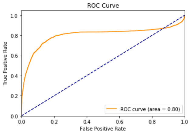
FIGURE 72 – Courbe ROC de New York pour 60 % des données avec l’algorithme utilisant le coefficient de Jaccard pour la prédiction des arêtes
