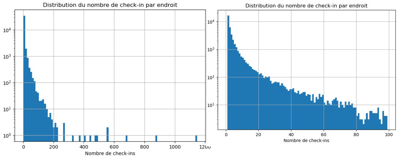
FIGURE 23 – Distribution du nombre d'entrées par endroit pour les 100 premières valeurs à New-York
