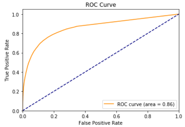
FIGURE 57 – Courbe ROC de Tokyo pour 35 % des données avec l’algorithme utilisant le coefficient de Jaccard pour la prédiction des arêtes
