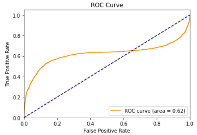
FIGURE 75 – Courbe ROC de Tokyo pour 35 % des données avec l’algorithme utilisant le coefficient de Jaccard pour la prédiction des arêtes
