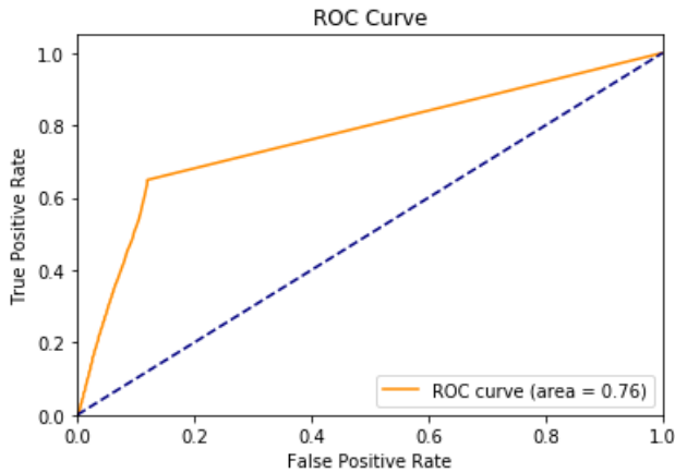
FIGURE 50 – Courbe ROC de New York pour 35 % des données avec l’algorithme utilisant le coefficient de Jaccard pour la prédiction des arêtes
