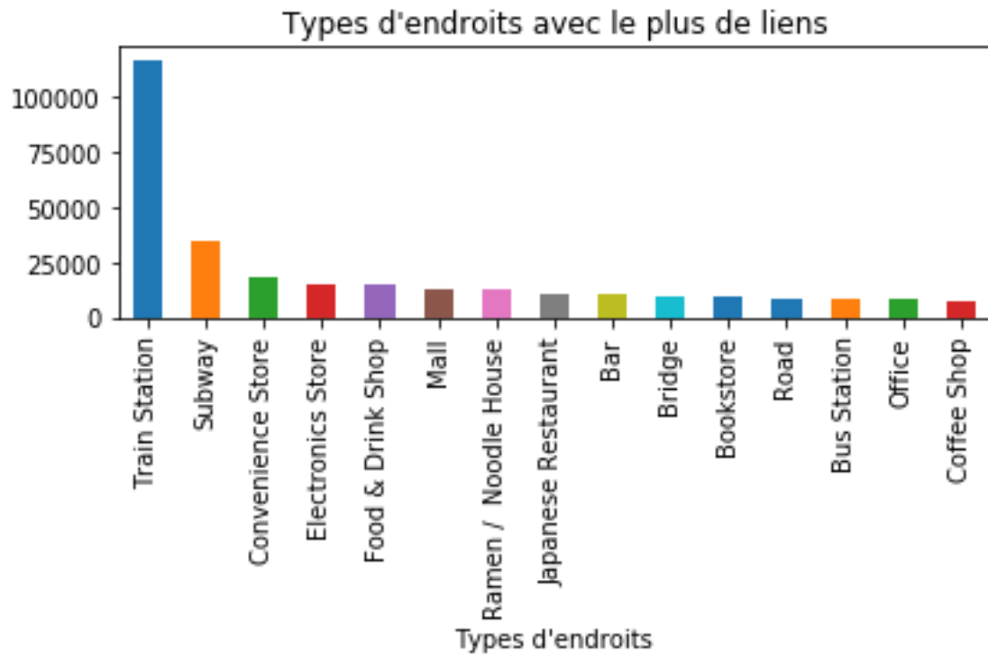
FIGURE 13 – Nombres de liens en fonction du type d'endroits à Tokyo
