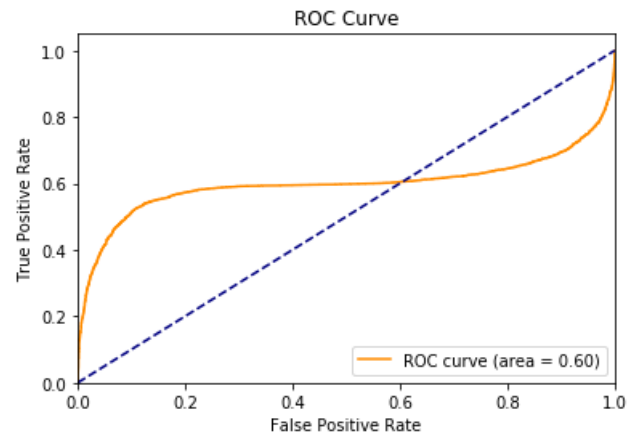
FIGURE 73 – Courbe ROC de Tokyo pour 60 % des données avec l’algorithme utilisant le coefficient de Jaccard pour la prédiction des arêtes
