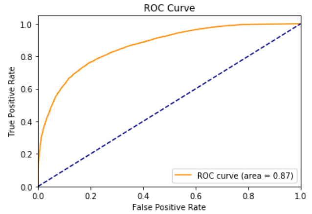
FIGURE 47 – Courbe ROC de Tokyo pour 85 % des données avec l’algorithme utilisant le coefficient de Jaccard pour la prédiction des arêtes
