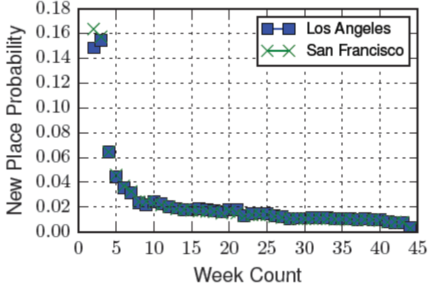
FIGURE 2 – Probabilité de découvrir un nouvel endroit sur le total d’endroits trouvés en fonction du nombre de semaines pour Los Angeles et San Francisco et ce à partir de la deuxième semaine. Source : [21]
