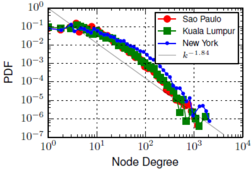
FIGURE 8 – Distribution de la densité de probabilité des degrés des noeuds sur une période de temps pour 3 villes et le comportement linéaire qui leur est associé. Source : [21]
