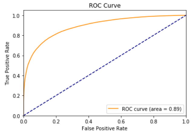
FIGURE 69 – Courbe ROC de Tokyo pour 35 % des données avec l'algorithme utilisant le coefficient de Jaccard pour la prédiction des arêtes
