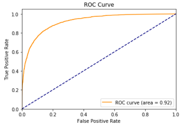
FIGURE 59 – Courbe ROC de Tokyo pour 85 % des données avec l'algorithme utilisant le coefficient de Jaccard pour la prédiction des arêtes
