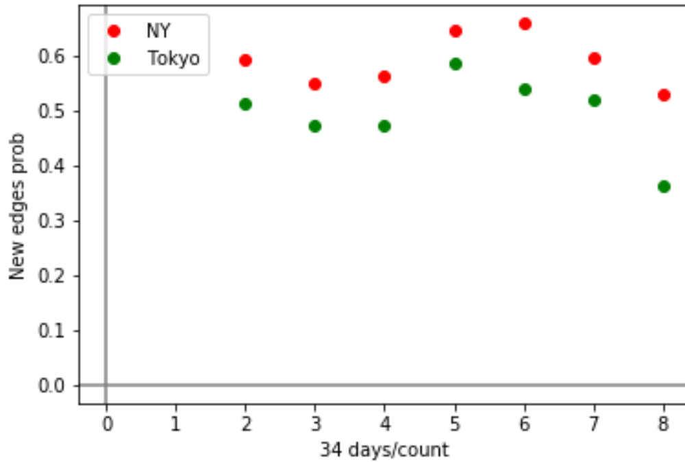
FIGURE 40 – Probabilité de découvrir une nouvelle arête entre deux endroits entre deux périodes de temps pour New York et Tokyo
