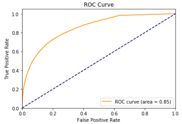
FIGURE 49 – Courbe ROC de Tokyo pour 60 % des données avec l’algorithme utilisant le coefficient de Jaccard pour la prédiction des arêtes
