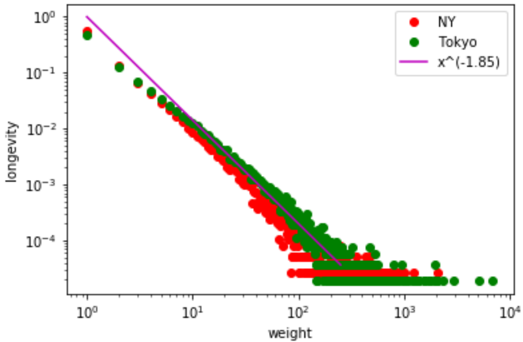
FIGURE 37 – Répartition des arêtes en fonction de leur poids pour la ville de New York.
