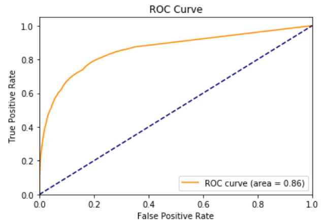
FIGURE 63 – Courbe ROC de Tokyo pour 35 % des données avec l’algorithme utilisant le coefficient de Jaccard pour la prédiction des arêtes
