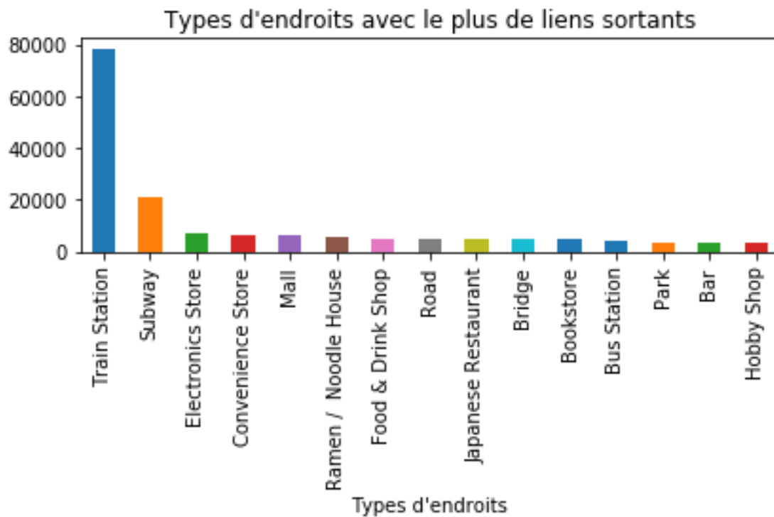
FIGURE 15 – Nombres de liens sortants en fonction du type d'endroits à Tokyo
