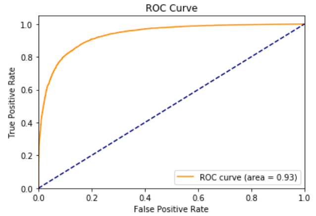
FIGURE 53 – Courbe ROC de Tokyo pour 85 % des données avec l'algorithme utilisant le coefficient de Jaccard pour la prédiction des arêtes
