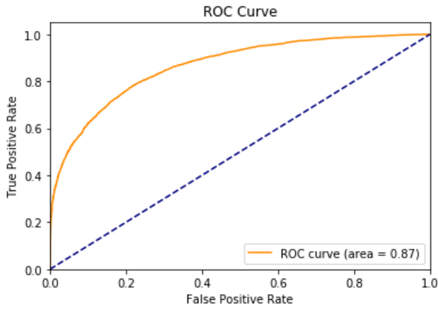
FIGURE 64 – Courbe ROC de New York pour 85 % des données avec l’algorithme utilisant le coefficient de Jaccard pour la prédiction des arêtes
