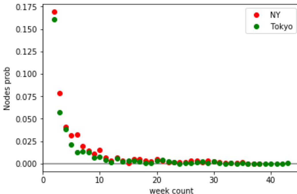
FIGURE 39 – Probabilité de découvrir un nouvel endroit sur le total d’endroits trouvés en fonction du nombre de semaines pour New York et Tokyo
