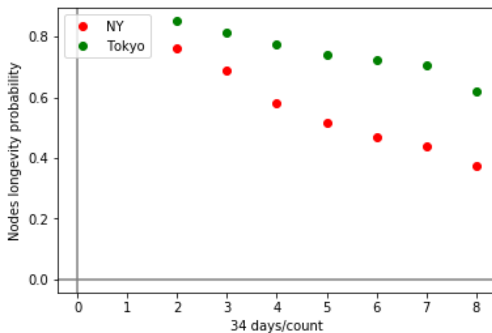
FIGURE 45 – Persistance des arêtes au fur est à mesure du temps
