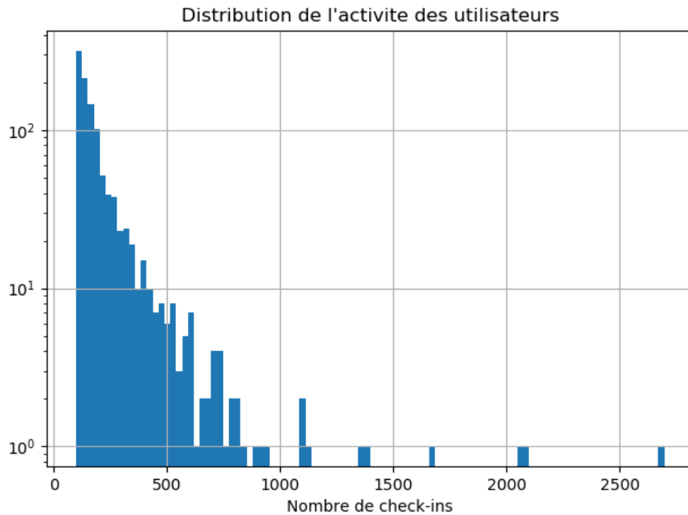
FIGURE 20 – Densité de répartitions du nombre de check-ins par utilisateur
