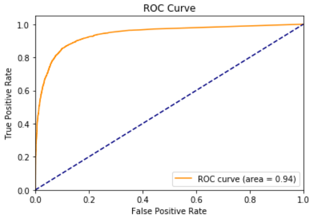
FIGURE 52 – Courbe ROC de New York pour 85 % des données avec l'algorithme utilisant le coefficient de Jaccard pour la prédiction des arêtes
