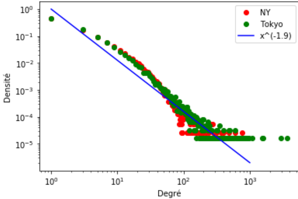
FIGURE 25 – Densité des noeuds en fonction de leur degré
