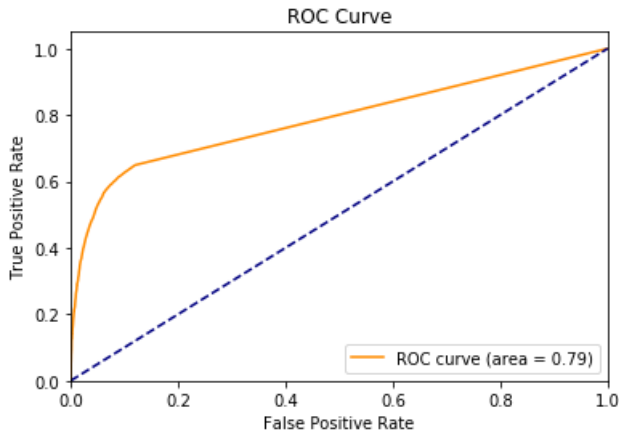
FIGURE 56 – Courbe ROC de New York pour 35 % des données avec l’algorithme utilisant le coefficient de Jaccard pour la prédiction des arêtes
