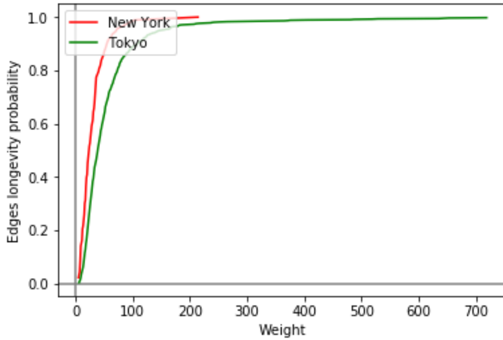
FIGURE 34 – Persistance des arêtes en fonction du poids de celles-ci sur la totalité des périodes de temps
