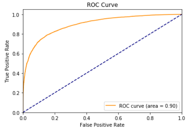
FIGURE 65 – Courbe ROC de Tokyo pour 85 % des données avec l’algorithme utilisant le coefficient de Jaccard pour la prédiction des arêtes
