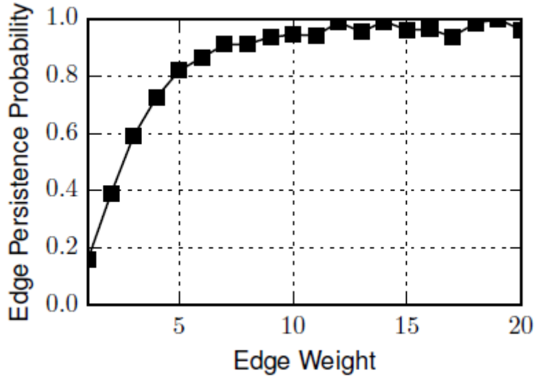
FIGURE 5 – Probabilité qu’une arête déjà présente dans les temps précédents réapparaisse dans le temps suivant en fonction du poids de cet arête. Source : [21]
