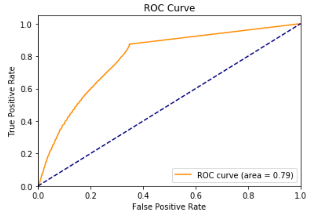
FIGURE 51 – Courbe ROC de Tokyo pour 35 % des données avec l’algorithme utilisant le coefficient de Jaccard pour la prédiction des arêtes
