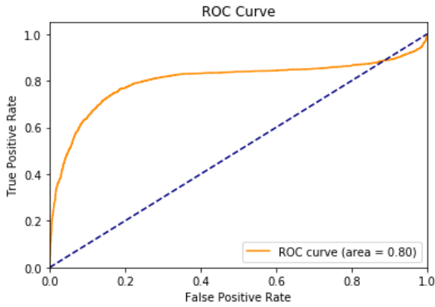
FIGURE 74 – Courbe ROC de New York pour 35 % des données avec l’algorithme utilisant le coefficient de Jaccard pour la prédiction des arêtes
