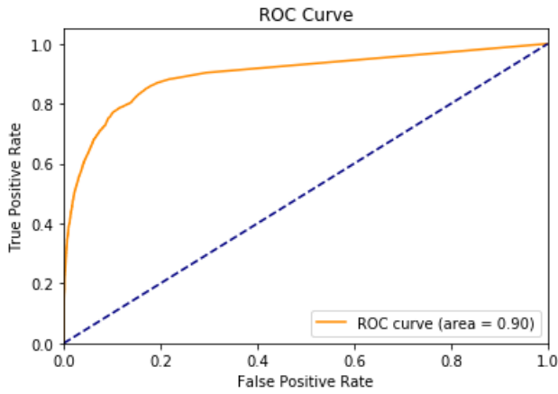
FIGURE 60 – Courbe ROC de New York pour 60 % des données avec l’algorithme utilisant le coefficient de Jaccard pour la prédiction des arêtes
