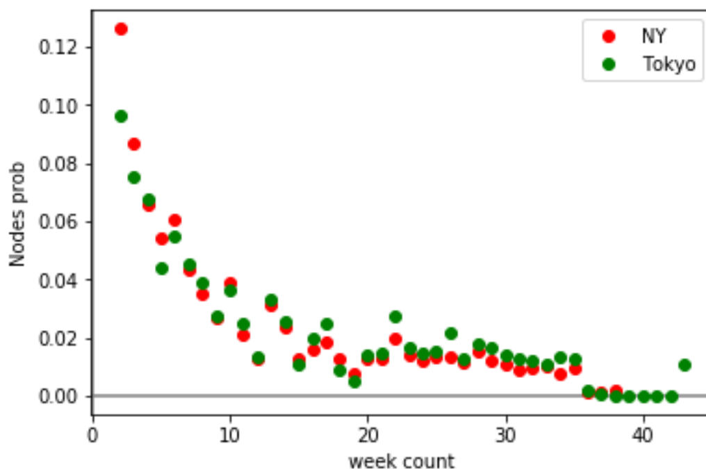
FIGURE 29 – Probabilité de découvrir un nouvel endroit sur le total d’endroits trouvés en fonction du nombre de semaines pour New York et Tokyo
