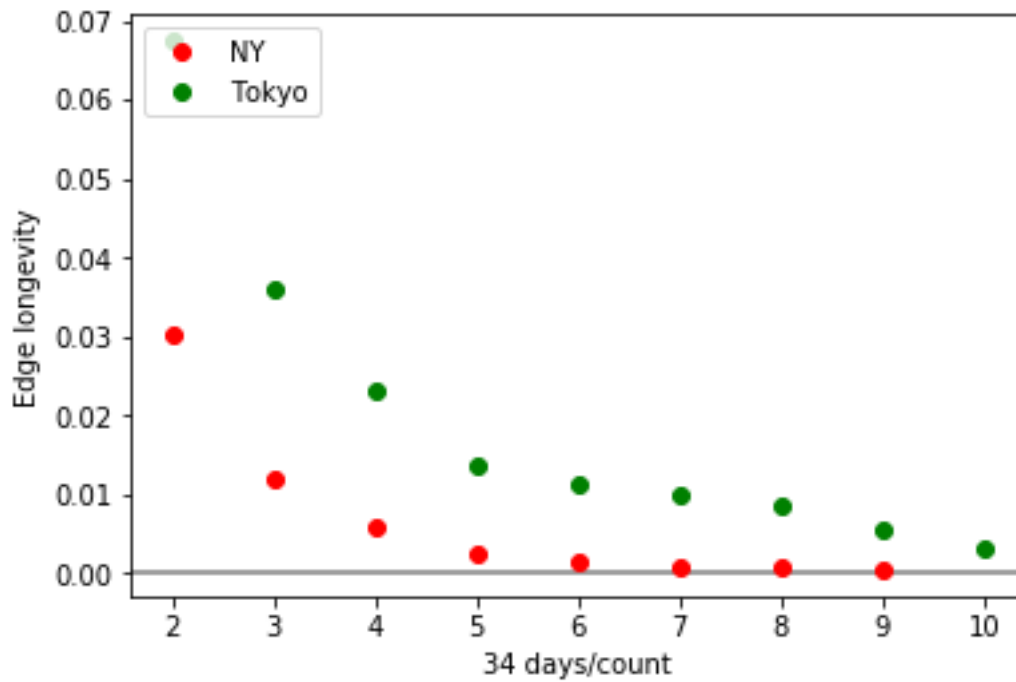
FIGURE 32 – Persistance des arêtes au fur et à mesure du temps
