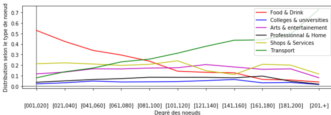
FIGURE 19 – Distribution du type de noeud en fonction de leur degré au sein de la ville de Tokyo
