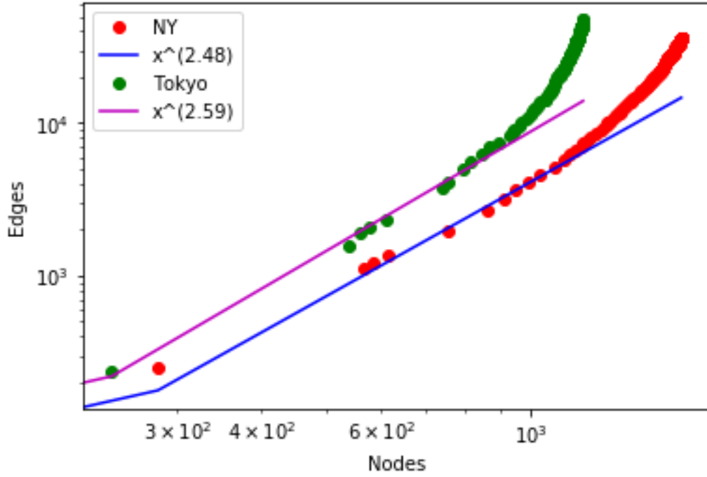
FIGURE 38 – Nombres de noeuds en fonction du nombre d'arêtes
