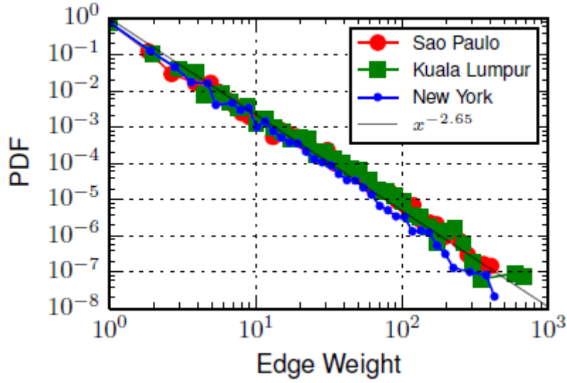
FIGURE 9 – Distribution de la densité de probabilité du poids des arêtes sur une période de temps pour 3 villes et le comportement linéaire qui leur est associé. Source : [21]
