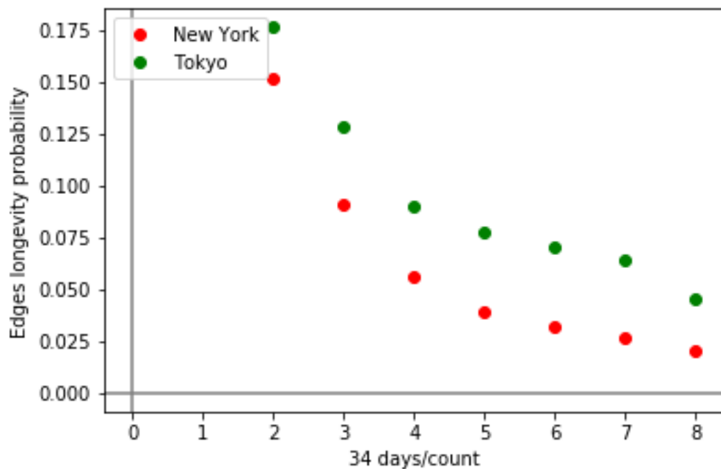
FIGURE 42 – Persistance des arêtes au fur et à mesure du temps
