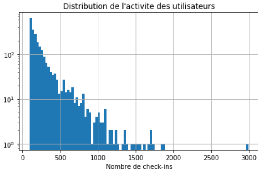
FIGURE 21 – Densité de répartition du nombre de check-ins par utilisateur
