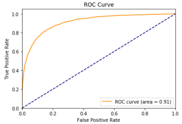
FIGURE 61 – Courbe ROC de Tokyo pour 60 % des données avec l’algorithme utilisant le coefficient de Jaccard pour la prédiction des arêtes
