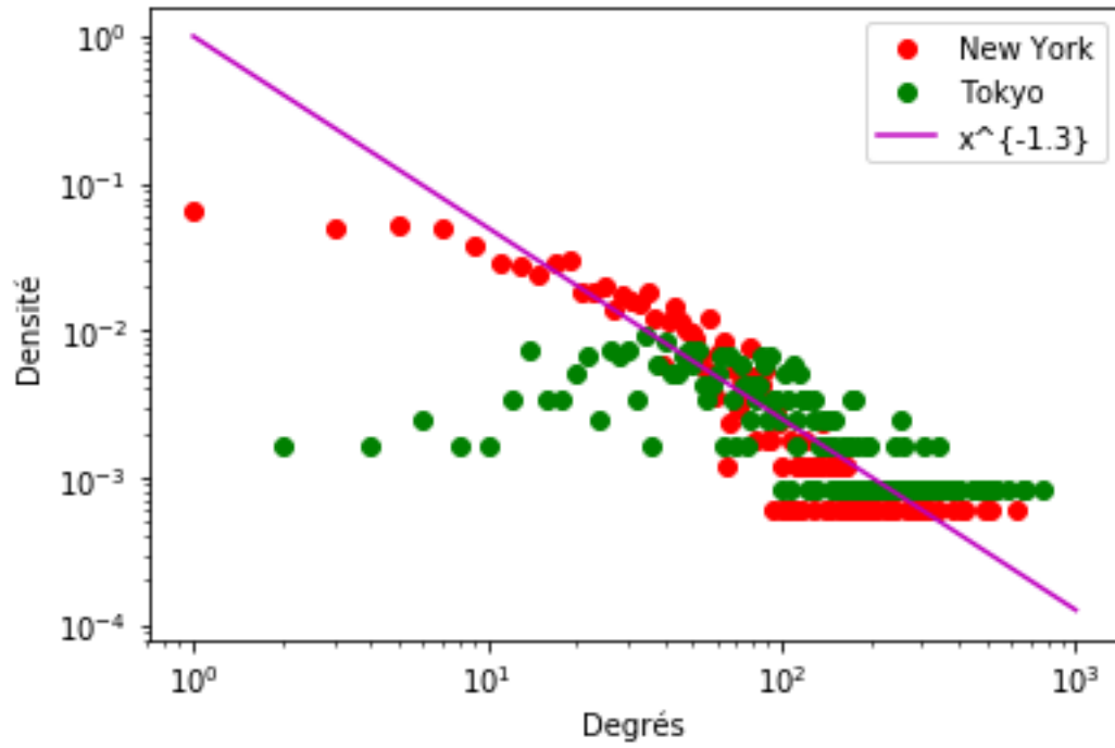
FIGURE 36 – Densité des noeuds en fonction de leur degré
