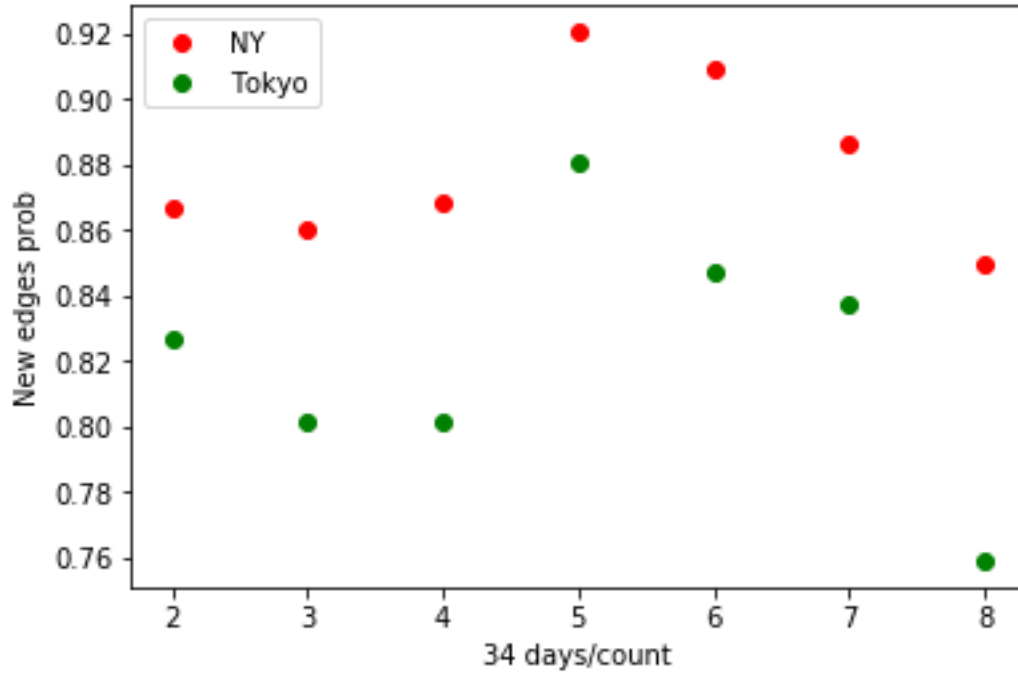
FIGURE 30 – Probabilité de découvrir une nouvelle arête entre deux endroits entre deux périodes de temps pour New York et Tokyo
