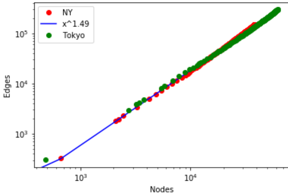
FIGURE 28 – Nombres de noeuds en fonction du nombre d'arêtes
