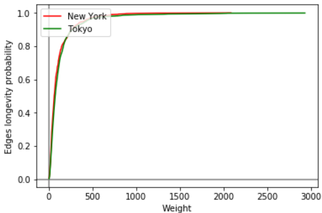
FIGURE 44 – Persistance des arêtes en fonction du poids de celles-ci sur la totalité du temps
