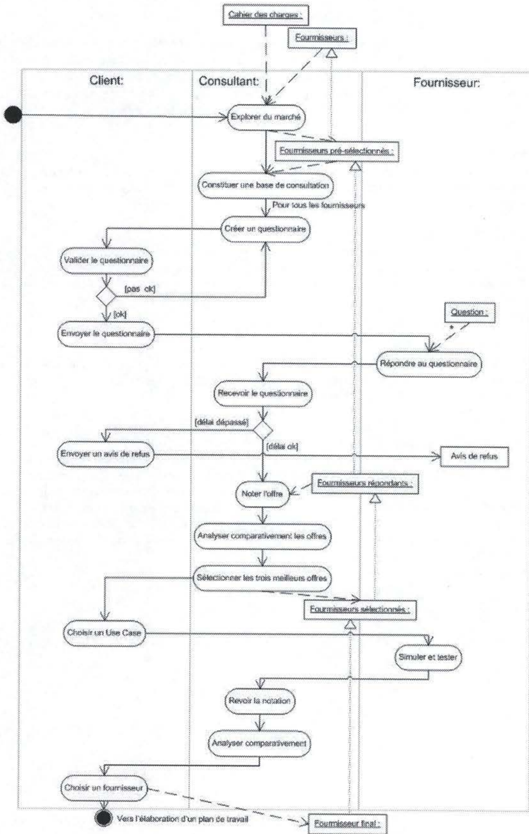
Figure 44 – Diagramme d'activités du processus « Appel Offres »
