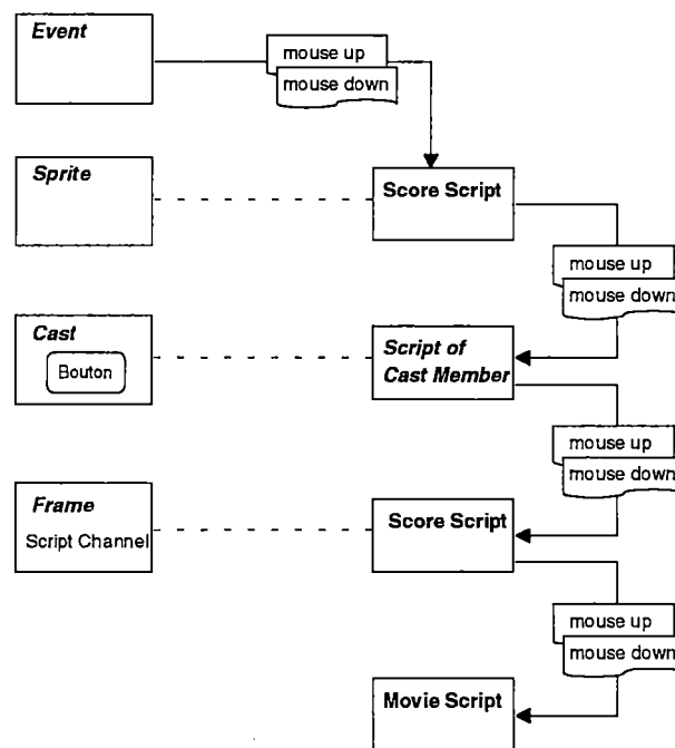
Figure 3.5. Le diagramme de passage des messages.
