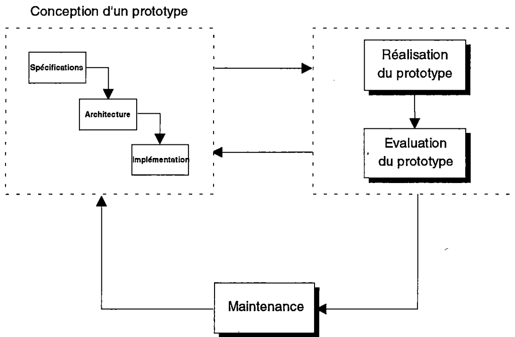
Figure 6.2 Un modèle de prototypage incrémental actualisé.
