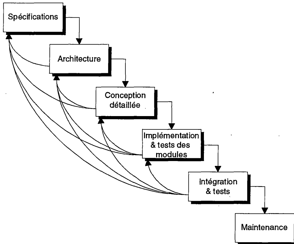
Figure 6.1 Le modèle de la cascade.
