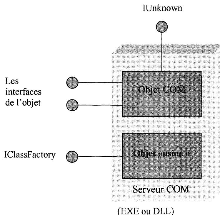
Figure 3.5. Un serveur COM.
