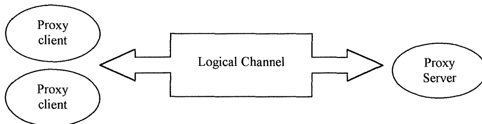
5.5. Architecture client-serveur.
