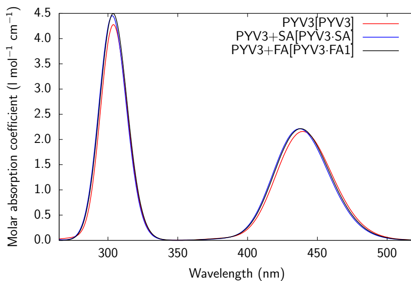
(b) Keto.
