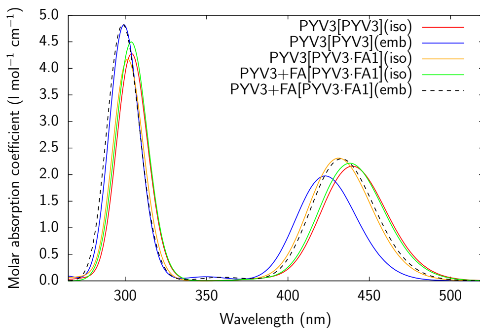
(b) Keto.
