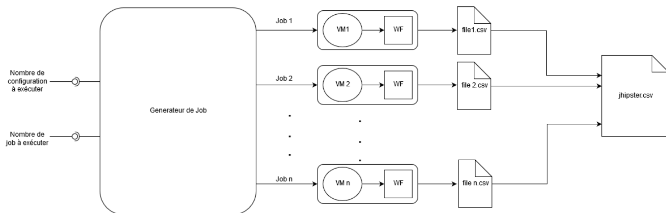
FIGURE 3.12 – Exécution du workflow sur IGRIDA
