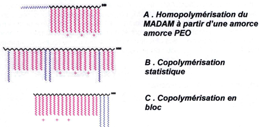
Figure III.3 : Représentation schématique des trois familles de polymères avec PEO synthétisées par le SMPC à l'UMH.
