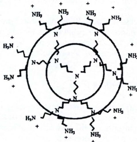
Figure 1.8 : Structure d'un dendrimère polyamidoaminé (PANAM) (Mumper et al, 1999)
