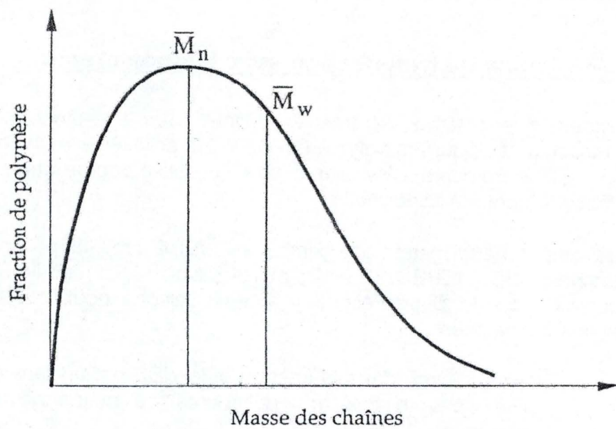
Figure III.2 : Distribution des masses moléculaires avec les moyennes en nombre \bar{M}_n et en poids \bar{M}_w
