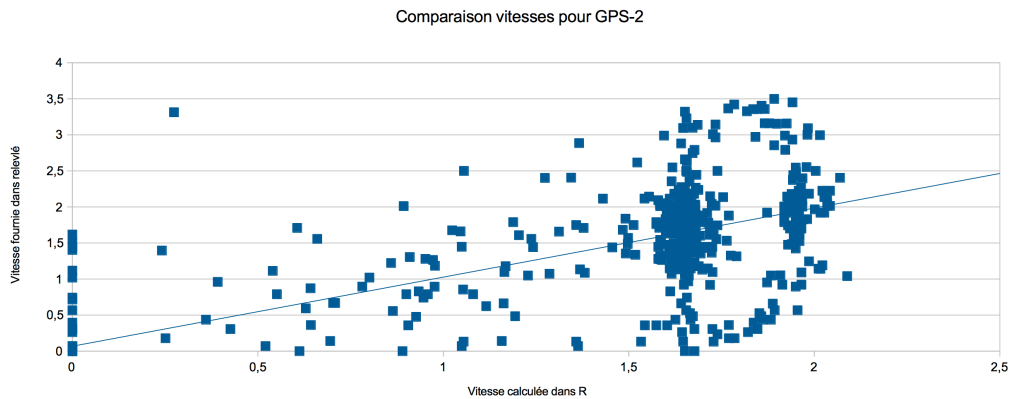
FIGURE 4.14 – Vitesse GPS-2 en fonction de la vitesse dans le fichier – Courbe de comparaison entre la vitesse disponible dans le fichier et la vitesse GPS-2 calculée dans R par la méthode Haversine.
