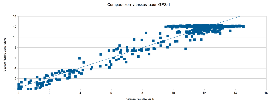
FIGURE 4.5 – Vitesse GPS-1 en fonction de la vitesse dans le fichier – Courbe de comparaison entre la vitesse disponible dans le fichier et la vitesse GPS-1 calculée dans R par la méthode Haversine.
