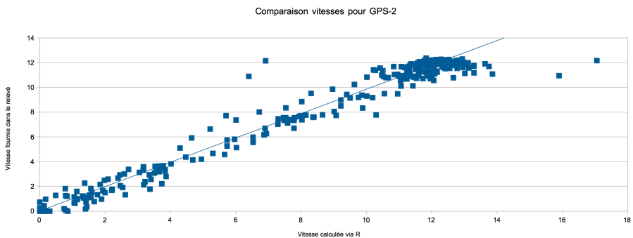
FIGURE 4.6 – Vitesse GPS-2 en fonction de la vitesse dans le fichier – Courbe de comparaison entre la vitesse disponible dans le fichier et la vitesse GPS-2 calculée dans R par la méthode Haversine.
