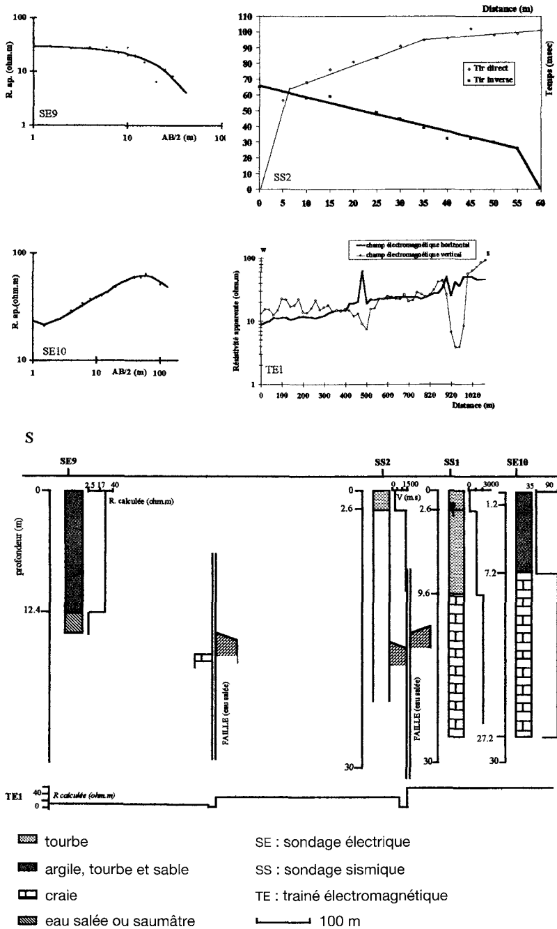
Figure 3 Essais géophysiques et leur traduction géologique le long du trainé électromagnétique TE1. Geophysical tests and their geological interpretation along electromagnetic profile TE1.
