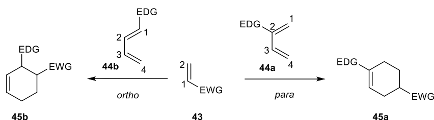
SCHEMA 1.3-6. La régiosélectivité ortho et para de la réaction de Diels-Alder entre un diène 44 substitué par un EDG et un diénophile 43 substitué par un EWG.
