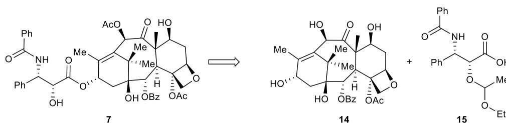
SCHEMA 1.1-3. Rétrosynthèse du Taxol® ( 7 ) à partir de la 10-déacétylbaccatine III ( 14 ) et le composé 15 . 17
