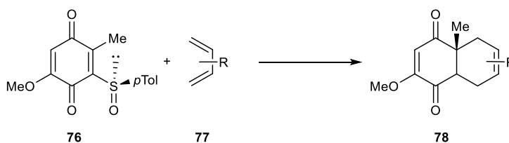
FIGURE 2.1-1. Réaction de Diels-Alder entre la sulfinylquinone 76 et différents diènes 77 pour la première étape de synthèse de la momilactone A ( 23a ).
