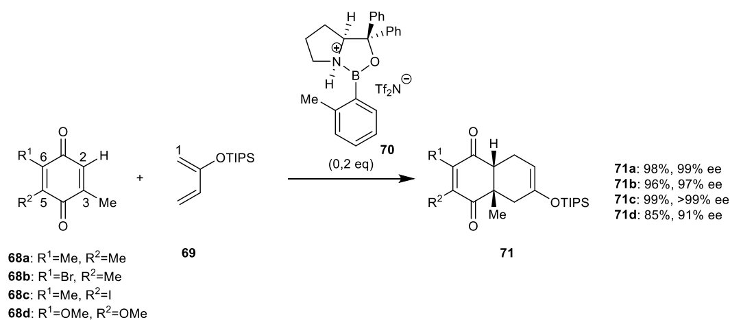
SCHEMA 1.3-10. Réaction asymétrique de Diels-Alder développée par Corey entre les différentes quinones 68 trisubstituées et le butadiène 69 catalysée par l'oxazaborolidinium 70 (0,2 eq). 58
