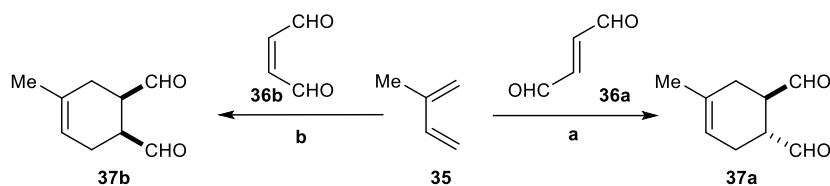
SCHEMA 1.3-3. La stéréospécificité de la réaction de Diels-Alder selon deux cas : a . Le diénophile 36a avec une relation trans donne le produit racémique 37a avec une configuration trans ; b . Le diénophile 36b avec une relation cis donne le produit racémique 37b avec une configuration cis .
