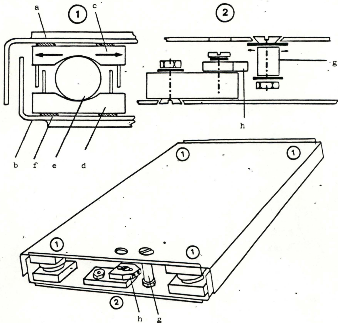
Fig. 5-4 ; plateau capteur de vibrations.
