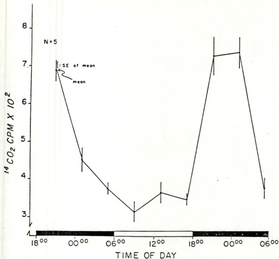
Fig I-3. Variation circadienne de l'activité de l'ornithine décarboxylase au niveau du foie d'un rat mâle. L'activité a été déterminée par la mesure de la libération de \text{CO}_2 à partir d'ornithine I- \text{C} .
