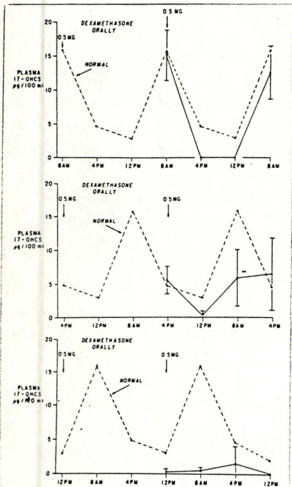
FIG. 2. Influence du moment de l'administration de dexaméthasone 0.5 mg per os sur les variations nyctémérales des concentrations plasmatiques des 17-hydroxycorticoïdes.
