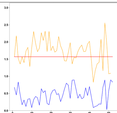
Figure 47 Changements de direction des instances en haute dimension du dataset COVID
