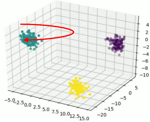
Figure 16 Etat final des instances et trajectoire (nuage vert) de Blob_MCu
