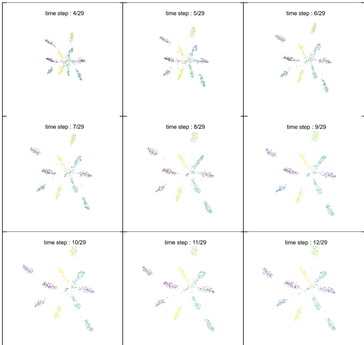
Figure 78 Animation d'une succession de projections générées par le dynamic t-SNE pénalisant les accélérations sur le dataset SVHN
