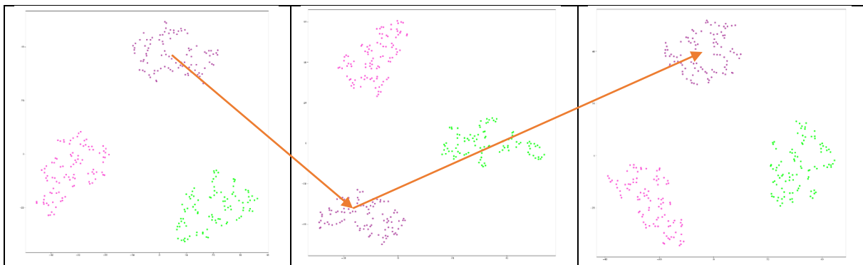
Figure 5 Le t-SNE avec des données temporelles. Les 3 images correspondent à trois time steps consécutifs
