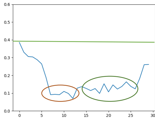
Figure 266 Détection des deux collisions inter-cluster du dataset Blob_MRUA à l'aide du temporal AUClogRNX avec pour time step de référence : 0/29 (TCP+)
