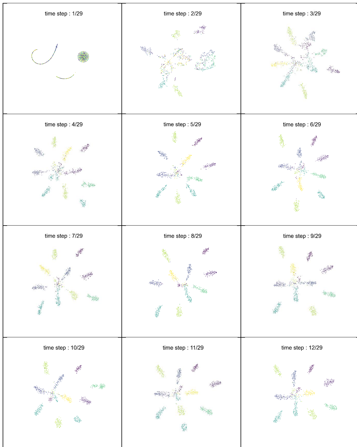
Figure 6 Animation d'une succession de t-SNE sur le dataset SVHN
