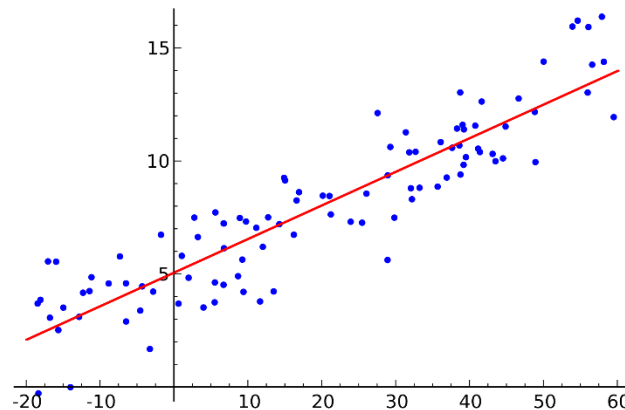
Figure 1 Régression linéaire sur un nuage de points bi-dimensionnel [1]
