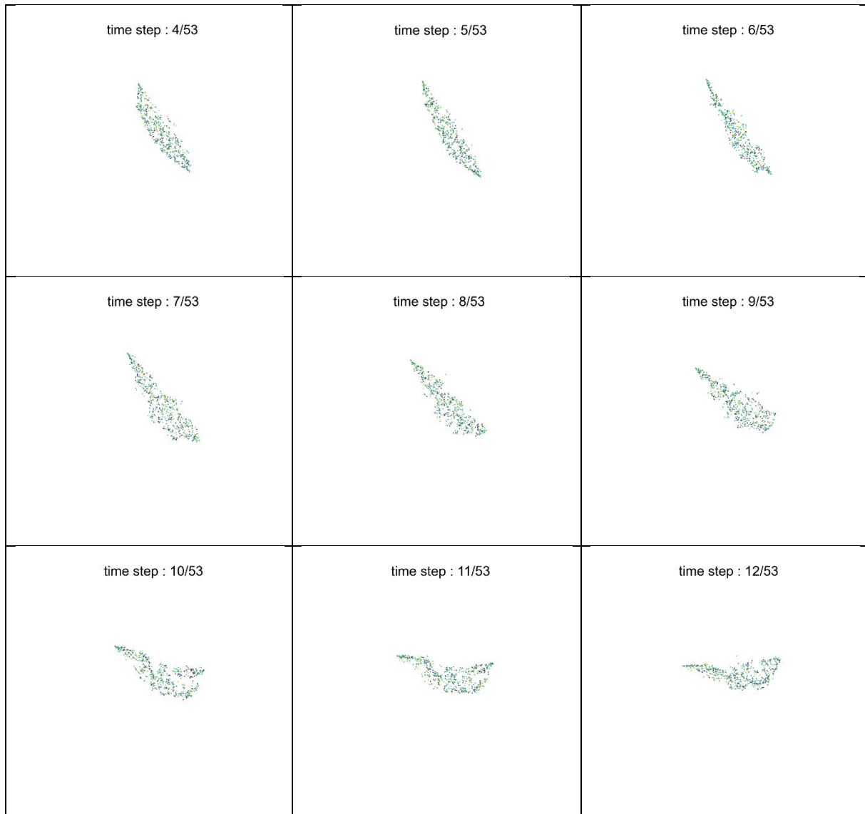
Figure 79 Animation d'une succession de projections générées par le dynamic t-SNE pénalisant les accélérations sur le dataset du Covid
