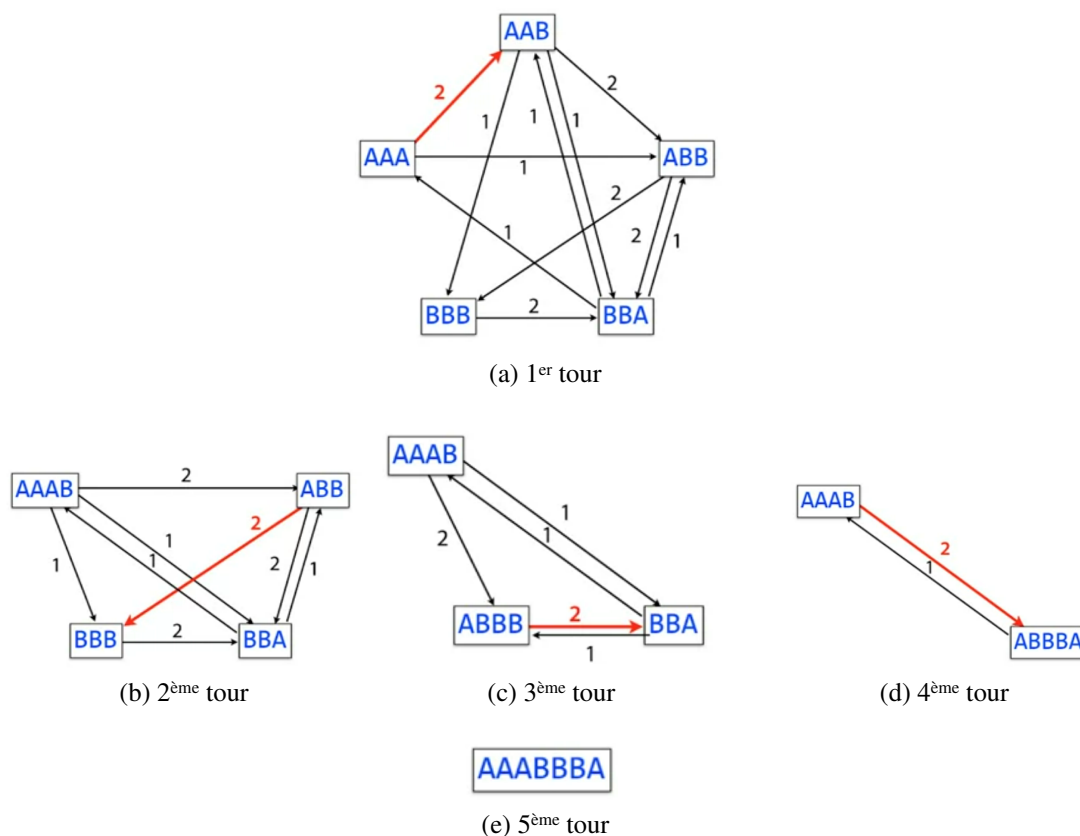
FIGURE 2.4.3 – Itérations de l'algorithme glouton
