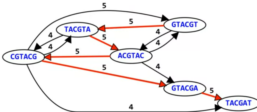
FIGURE 2.4.2 – Graphe de chevauchement
