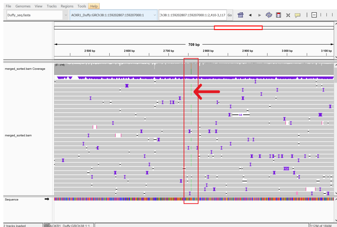
FIGURE 4.2.1 – Visualisation des reads alignés sur le génome de référence Duffy avec le logiciel IGV. La flèche montre une mutation à la position 2 758 visible sur l'ensemble des reads
