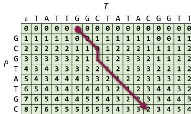
FIGURE 2.1.1 – Trace de la distance d'édition
