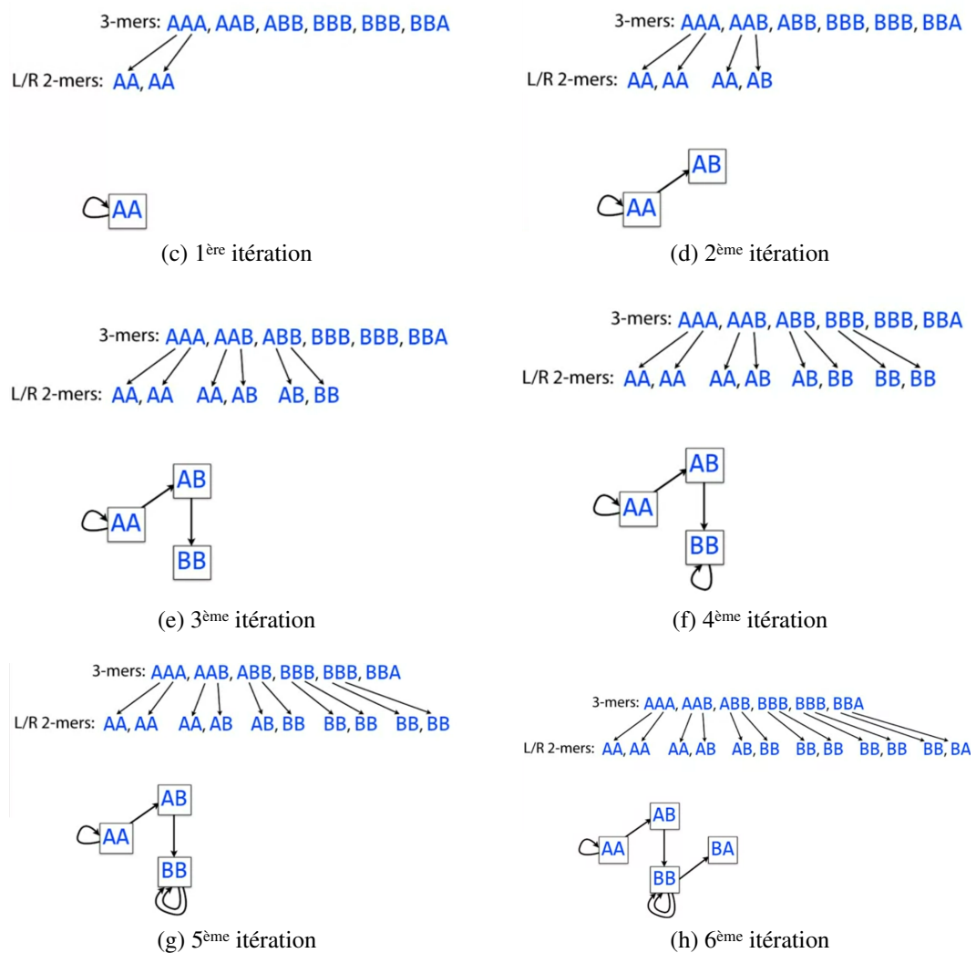
FIGURE 2.4.4 – Illustration des étapes lors de la construction d'un graph de De Bruijn
