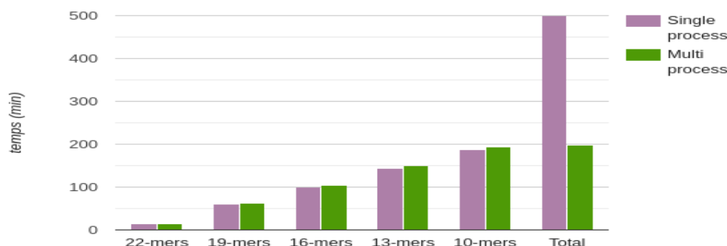
FIGURE 3.2.11 – Comparaison du temps d'exécution total entre le single processing et multiprocessing pour le calcul des 22-mers, 19-mers, 16-mers, 13-mers et 10-mers du génome humain
