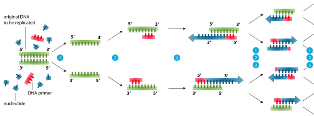
FIGURE 3.1.1 – Cycle de PCR et rôle des amorces [17] avec la représentation des phases de dénaturation (1) qui permet de séparer les brins d'ADN, d'hybridation (2) où l'amorce vient s'accrocher sur le brin d'ADN complémentaire, d'élongation (3) où l'ADN se multiplie
