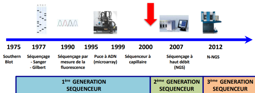
FIGURE 1.4.2 – Techniques de séquençage d'ADN par génération : la couleur bleue pour la 1ère génération de séquençage qui est marquée par un début d'automatisation des séquençages avec la technique de Sanger qui est une méthode par synthèse enzymatique sélective. En vert, la 2ème génération de séquençage , aussi appelée séquençage haut débit (HTS pour high-throughput sequencing) ou NGS pour next-génération, permettant l'augmentation du débit d'analyse de façon très importante passant de quelques milliers de paires de bases séquencées à plusieurs milliards. En orange, la 3ème génération de séquençage qui permet le séquençage direct de molécules uniques et rend ainsi superflu le marquage fluorescent ou d'autres étapes préparatoires spécifique [61].
