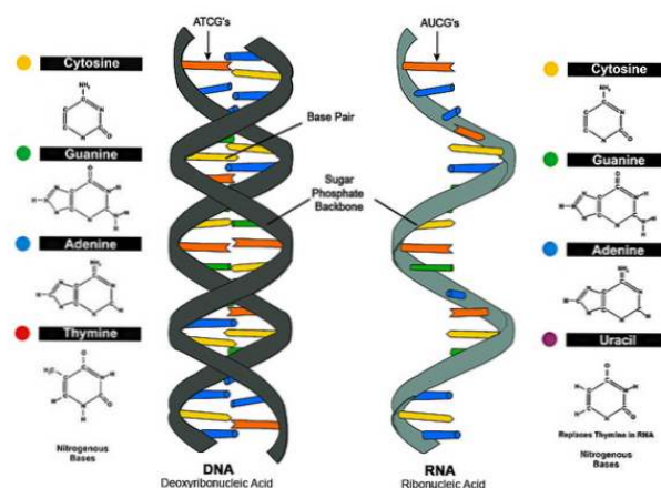
FIGURE 1.1.1 – Représentation d'une molécule d'ADN double brin (à gauche) et d'une molécule d'ADN simple brin (à droite) ainsi que de leurs bases nucléotidiques associées [20].
