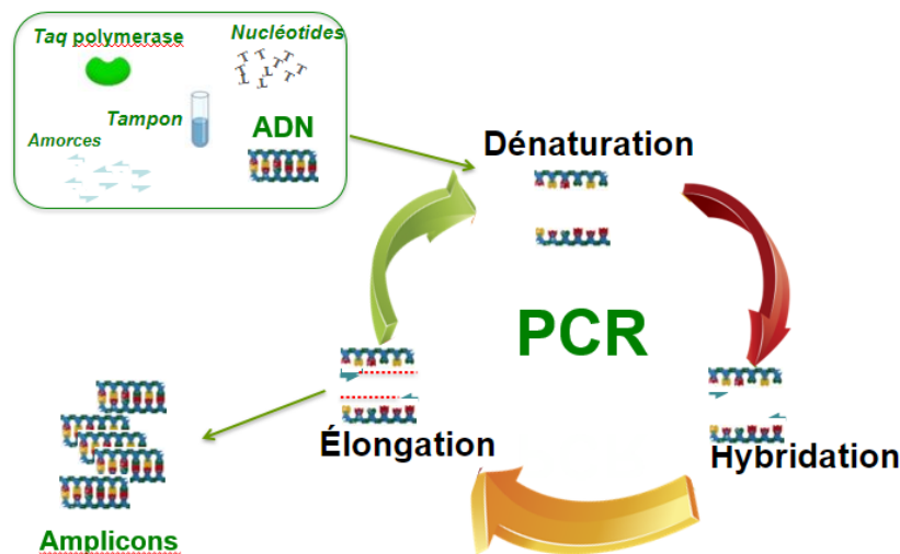
FIGURE 1.3.1 – Principe de la PCR : effectue un cycle passant par trois étapes principales. Chacun débute par l'étape de dénaturation lorsque les 2 brins de l'ADN se séparent par rupture des liaisons hydrogènes, pour obtenir des matrices simples brin. Ensuite dans l'étape d'hybridation, à 50°C-65°C, les amorces individuelles viennent s'accrocher sur ceux-ci. La dernière phase est l'élongation à 72°C, la taq polymérase se charge d'associer le nucléotide correspondant à son partenaire sur le brin guide. Courtesy of Prof. P. Bogaerts.
