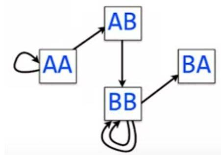
FIGURE 2.4.5 – Graphe de De Bruijn final après sa construction
