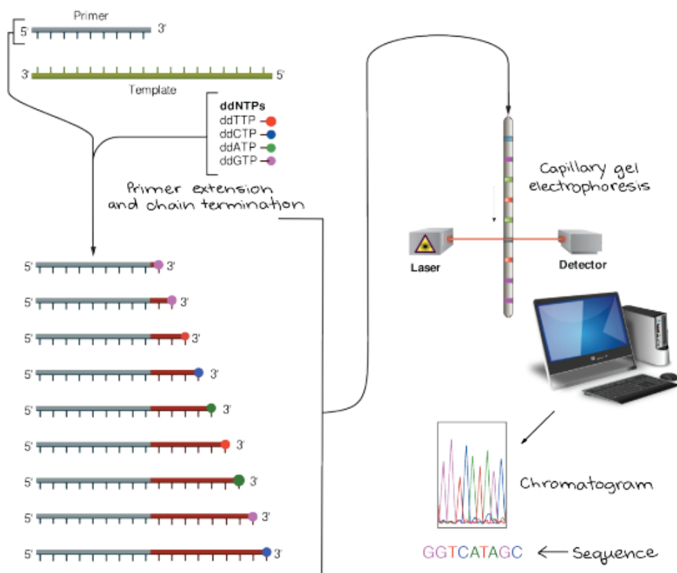
FIGURE 1.4.3 – Séquençage Sanger. Les fragments d'ADN synthétisés sont séparés en fonction de leur taille par électrophorèse sur gel et leur terminaison fluorescente est lue par le lecteur laser qui va identifier le ddNTP 2 correspondant [70].
