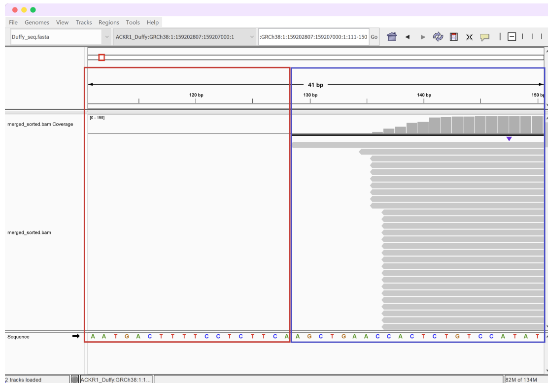
FIGURE 4.3.1 – Représentation IGV pour Duffy illustrant dans le cadre rouge une zone non-couverte par des alignements et en bleu une zone couverte par des alignements
