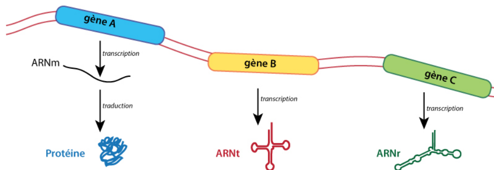
FIGURE 1.1.2 – Représentation d'un gène [50] : l'image représente un chromosome avec plusieurs gènes (qui sont une partie de cette information à un endroit précis). Le gène A est un exemple de transcription en ARNm (ARN messenger : qui est comme une copie, une molécule chargée de transmettre l'information codée dans le génome [67]) suivi d'une traduction en protéine qui va être une unité fonctionnelle. Dans le cas du gène B, c'est simplement une transcription en ARNt (ARN de transfert : qui est une courte molécule d'ARN, qui va associer à chaque codon un acide aminé parmi 20 possibles [39]). Dans le cas du gène C, c'est une transcription ARNr (ARN ribosomiale : constituant principal des ribosomes qui se charge d'assurer l'interaction de l'ARNm avec l'ARNt [8]) .
