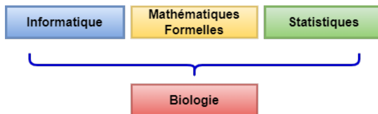
FIGURE 1.5.1 – Bio-informatique en temps que pluridisciplinarité scientifique
