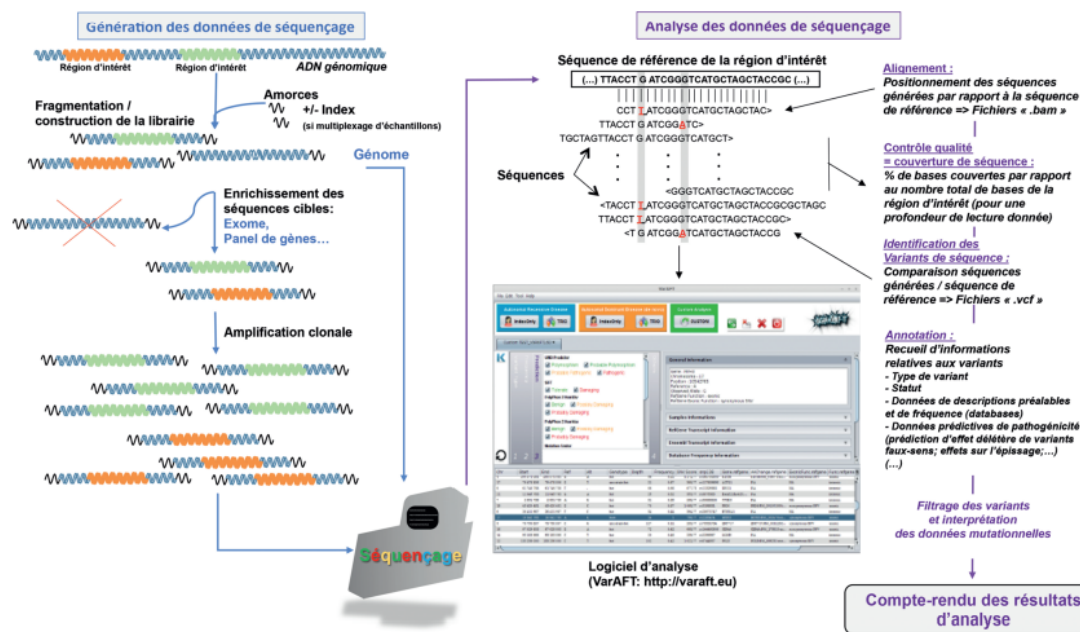
FIGURE 1.4.1 – Étapes du NGS qui se font principalement en trois phases. D'abord, la préparation des échantillons qui correspond en partie à la construction des librairies. Ensuite vient l'étape de séquençage proprement dite, effectuée par une technologie de NGS (Nanopore, illumina, etc). Enfin vient celle d'analyse ou les librairies séquencées sont alignées et annotées sur une séquence de référence pour obtenir un fichier .sam permettant d'effectuer d'autres processus comme l'illustre le schéma [44].
