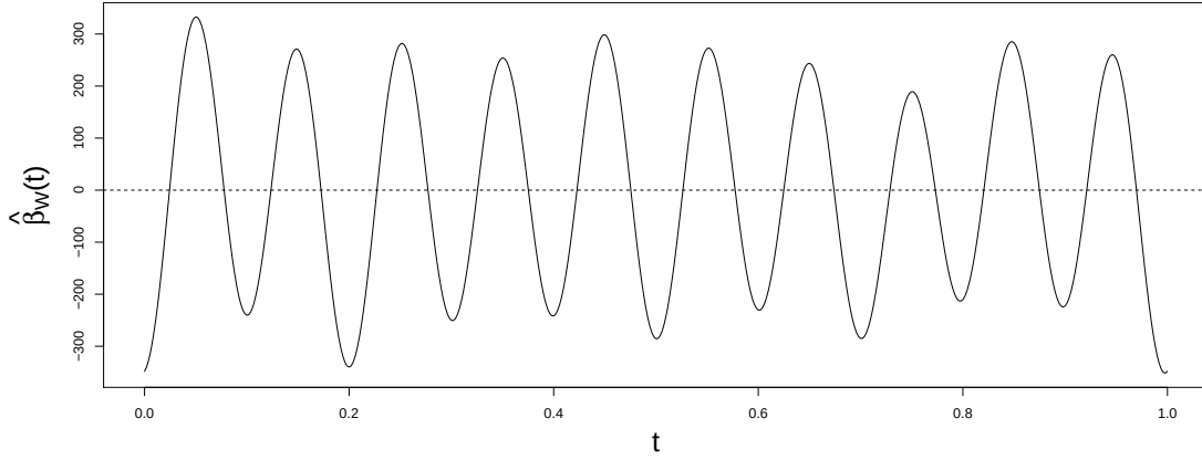
FIGURE 4.4 – Graphe pour le modèle 1 de l’estimateur naïf \hat{\beta}_W(t) obtenu grâce à la fonction fRegress en R . Le nombre de termes utilisés dans la base de la série de Fourier est de 25.
