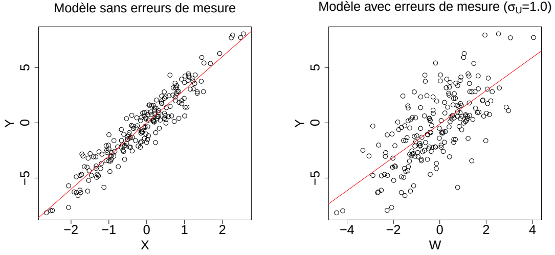
FIGURE 1.1 – Exemple d’une régression linéaire simple sans (à gauche) et avec erreurs de mesure (à droite), où \sigma_x^2 = 1 et \sigma_u^2 = 1 . La taille de l’échantillon vaut n = 1000 dans les deux cas et la valeur du paramètre sans erreur de mesure est \beta_x = 3 . Par (1.3), le paramètre du modèle avec erreurs de mesure vaut \beta_w = \beta_x/2 = 1.5 .
