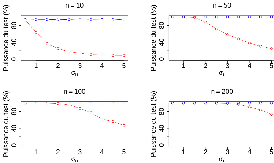
FIGURE 2.4 – Estimation de la puissance du test de significativité dans un modèle de régression avec erreurs de mesure pour la courbe en rouge et avec la correction apportée à l’estimateur par la méthode de la variable instrumentale pour la courbe en bleu, où n est la taille de l’échantillon. Le nombre de modèles utilisés pour estimer la puissance est de 1000 à chaque étape.
