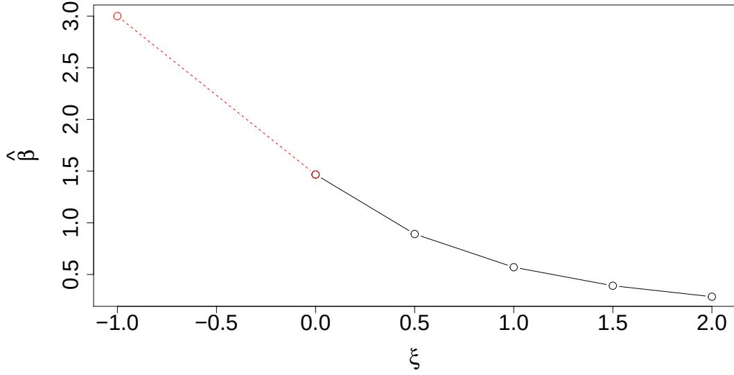
FIGURE 2.1 – Illustration de la méthode du SIMEX sur le modèle de la FIGURE 1.1. En noir, les valeurs obtenues pour \hat{\beta}_x en fonction des valeurs de \xi et en rouge, l'extrapolation que devrait donner idéalement l'algorithme du SIMEX en \xi = -1 , c'est-à-dire \beta_x = 3 .
