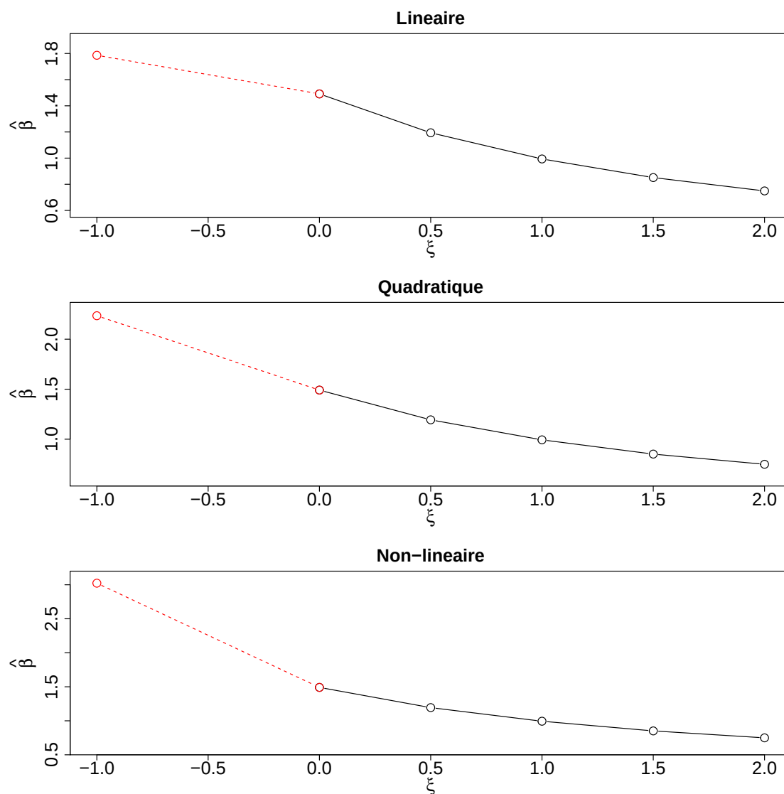
FIGURE 2.2 – Illustration des résultats obtenus par le SIMEX sur le modèle associé à la FIGURE 1.1. Le vrai paramètre \beta_x = 3 , la variance des erreurs de mesure \sigma_u^2 = 1 et la taille de l'échantillon n = 1000 . Les différents types d'extrapolation sont linéaire, quadratique et non-linéaire.
