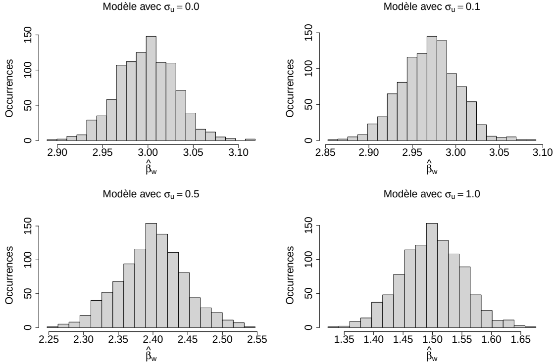
FIGURE 1.2 – Histogrammes des valeurs de \hat{\beta}_w d’une régression linéaire simple avec erreurs de mesure pour différentes valeurs de \sigma_u . La taille de l’échantillon vaut n = 1000 et le nombre d’itérations est de 1000. La valeur du paramètre sans erreur de mesure est \beta_x = 3 et \sigma_x^2 = 1 .
