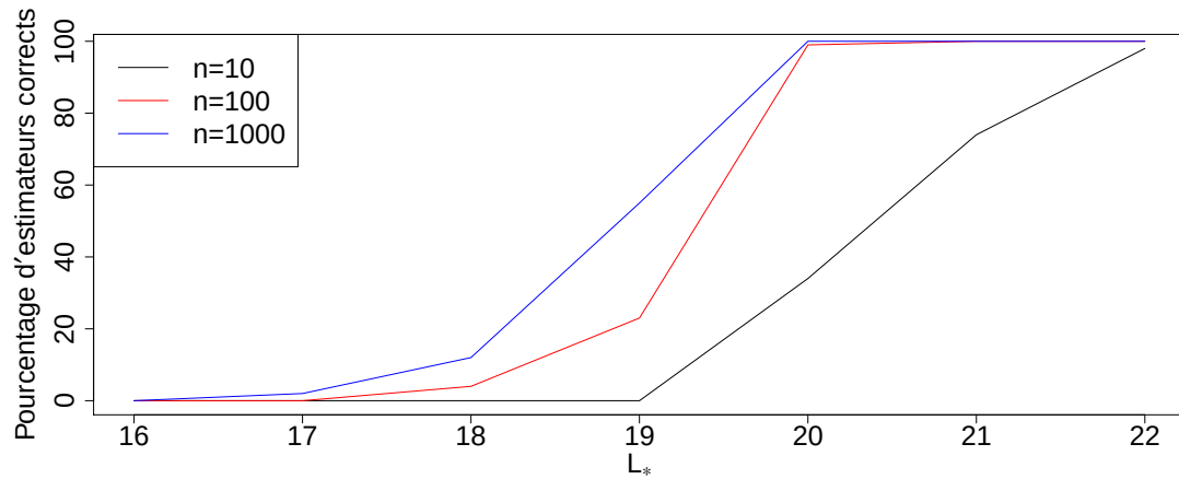
FIGURE 4.2 – Graphique du pourcentage d'estimateurs \hat{r}_{b,L_*} calculés par l'algorithme égaux à la vraie valeur du rang r en fonction de la taille de la sous-grille L_* .
