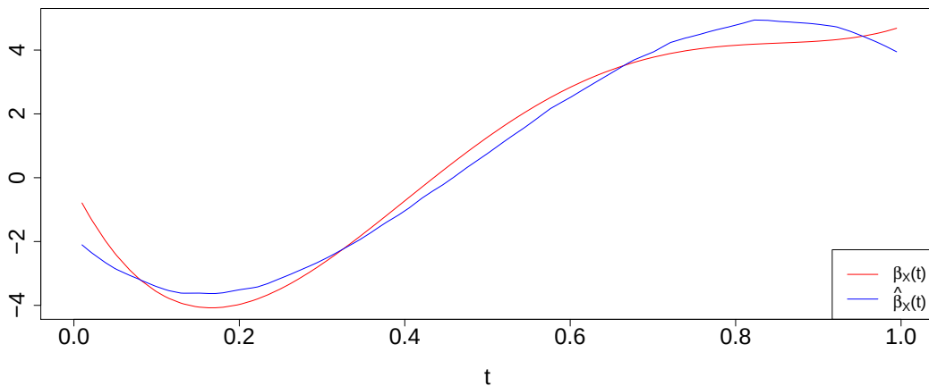
FIGURE 4.7 – Graphe pour le modèle 2 du vrai paramètre fonctionnel \beta_X(t) en rouge et de son estimateur \hat{\beta}_X(t) obtenu par l'algorithme corrigeant les effets de la présence d'erreurs de mesure en bleu.
