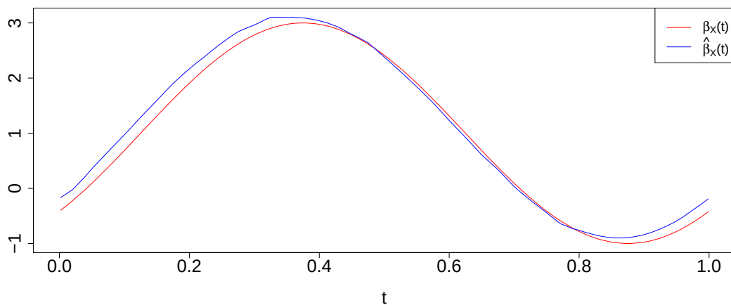
FIGURE 4.3 – Graphe pour le modèle 1 du vrai paramètre fonctionnel \beta_X(t) en rouge et de son estimateur \hat{\beta}_X(t) obtenu par l'algorithme corrigeant les effets de la présence d'erreurs de mesure en bleu.
