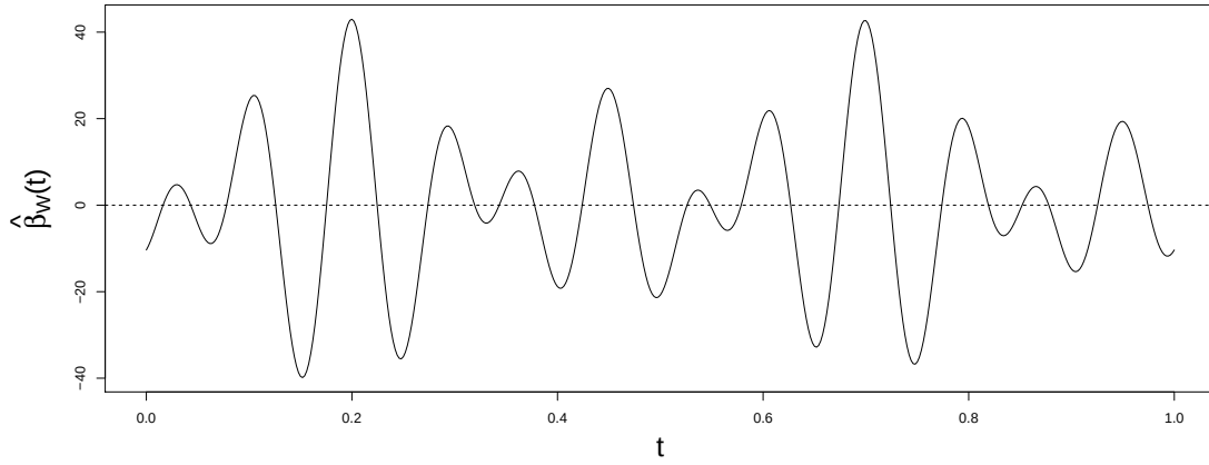
FIGURE 4.8 – Graphe pour le modèle 2 de l'estimateur naïf \hat{\beta}_W(t) obtenu grâce à la fonction fRegress en R . Le nombre de termes utilisés dans la base de la série de Fourier est de 25.
