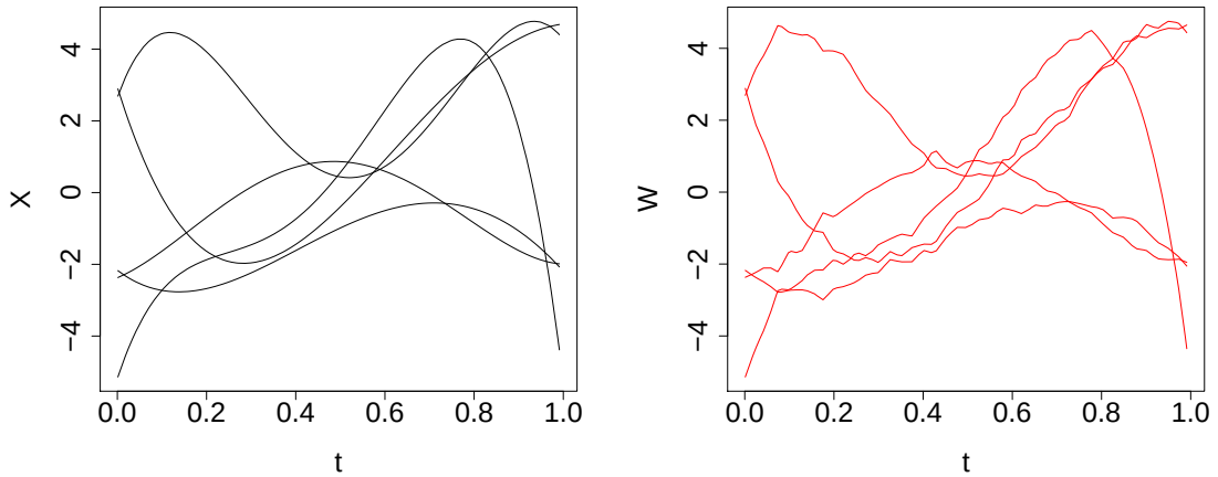
FIGURE 4.6 – Graphique des 5 premiers individus de l'échantillon pour la variable sans erreur de mesure X (à gauche) et des 5 individus correspondant pour la variable avec des erreurs de mesure W (à droite) dans le modèle 2.
