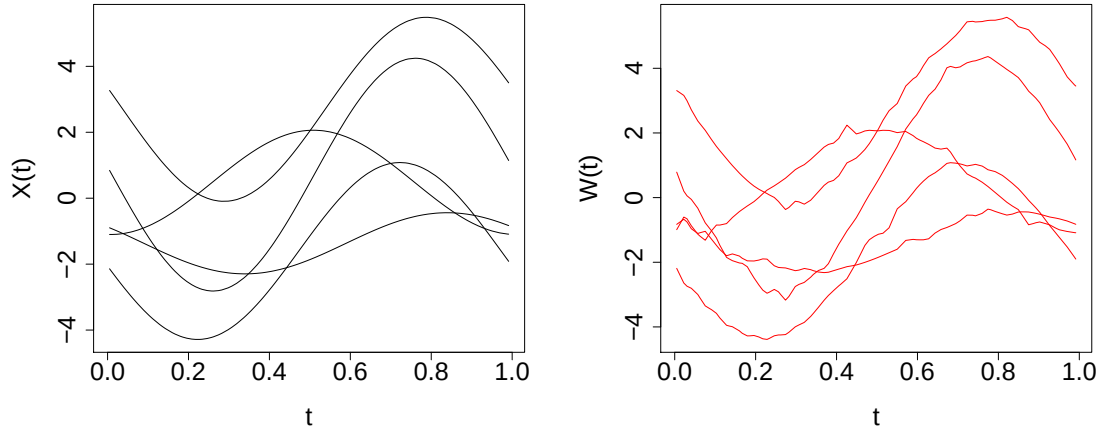
FIGURE 4.1 – Graphique des 5 premiers individus de l'échantillon pour la variable sans erreur de mesure X (à gauche) et des 5 individus correspondant pour la variable avec des erreurs de mesure W (à droite) dans le modèle 1.
