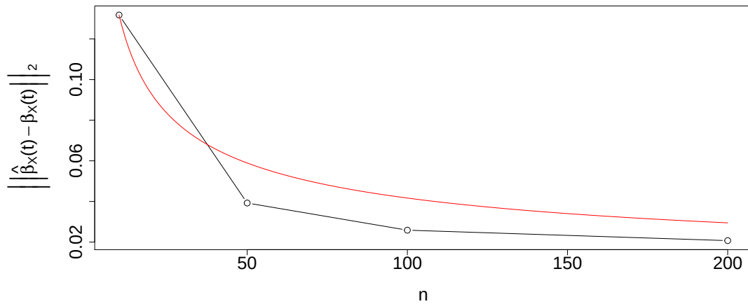
FIGURE 4.9 – Graphe pour le modèle 2 de l'erreur moyenne \|\cdot\|_2 entre le vrai paramètre fonctionnel \beta_X(t) et son estimateur \hat{\beta}_X(t) obtenu par l'algorithme en fonction de la taille de l'échantillon n en noir. La vitesse de convergence est \mathcal{O}(n^{-1/2}) (représentée en rouge). Le modèle a été généré 20 fois pour chaque valeur de n .
