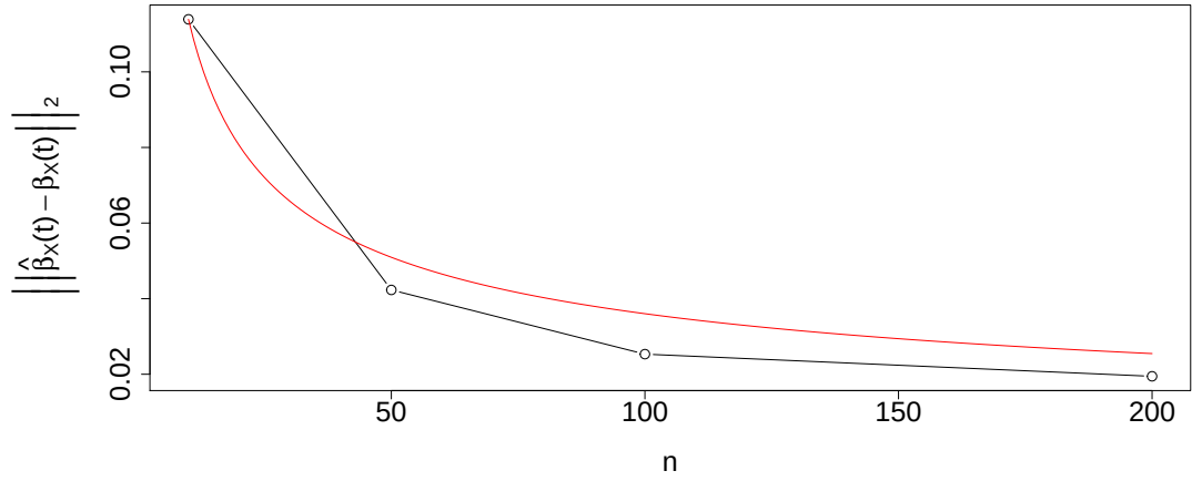
FIGURE 4.5 – Graphe pour le modèle 1 de l'erreur moyenne \|\cdot\|_2 entre le vrai paramètre fonctionnel \beta_X(t) et son estimateur \hat{\beta}_X(t) obtenu par l'algorithme en fonction de la taille de l'échantillon n en noir. La vitesse de convergence est \mathcal{O}(n^{-1/2}) (représentée en rouge). Le modèle a été généré 20 fois pour chaque valeur de n .
