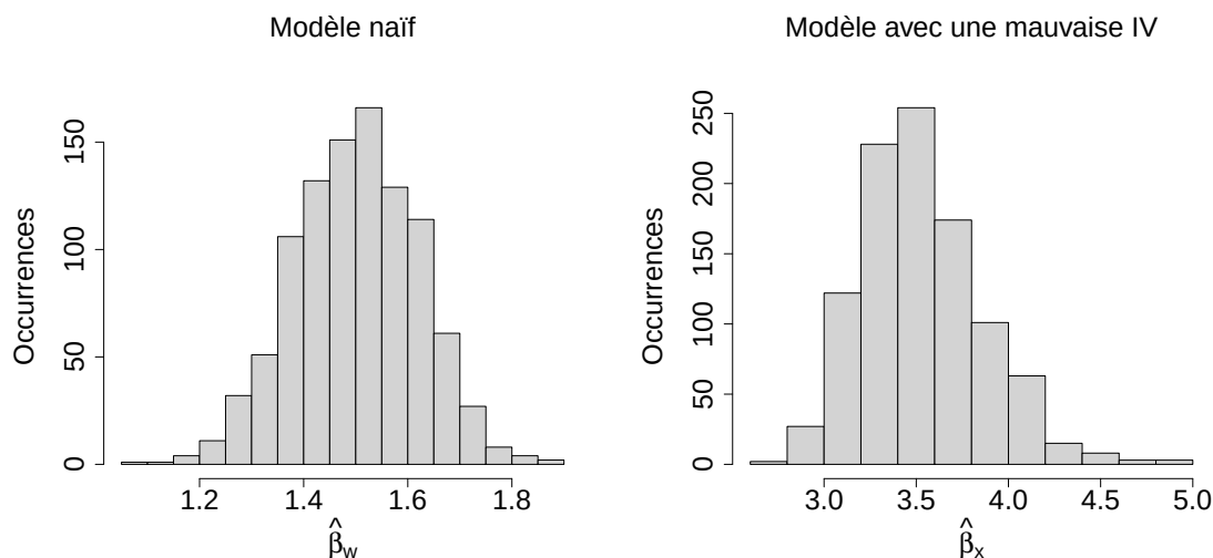
FIGURE 2.5 – Histogramme des valeurs de \hat{\beta}_w d’une régression linéaire simple avec erreurs de mesure où la correction via la méthode de la variable instrumentale se fait avec une variable ne respectant pas le critère \sigma_{t\varepsilon} = 0 . La vraie valeur du paramètre \beta_x = 3 .
