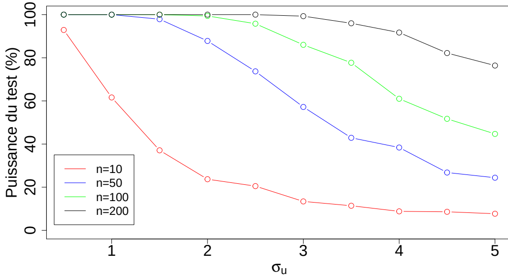
FIGURE 1.3 – Estimation de la puissance du test de significativité du coefficient associé au régresseur X dans un modèle de régression linéaire simple avec erreurs de mesure. L'échantillon est de taille n et les variables du modèle X \sim \mathcal{N}(0, 1) et \varepsilon \sim \mathcal{N}(0, 1) . Le vrai paramètre \beta_x = 3 et le nombre de modèles utilisés pour estimer la puissance est de 1000 à chaque étape.
