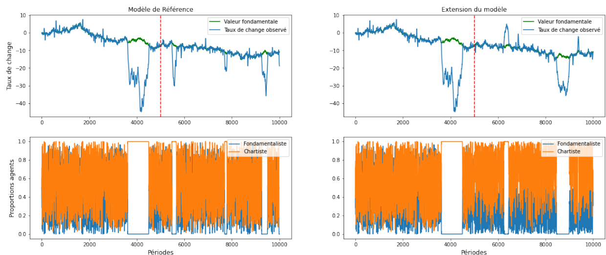
Figure 4.2.5 – Comparaison des dynamiques du taux de change et de la composition du marché pour l’extension (ajout des agents chartistes machine learner) et le modèle de référence - Exemple de périodes de stabilité et d’instabilité générées suite à l’ajout des agents. La ligne verticale rouge correspond à la période durant laquelle la nouvelle heuristique est introduite.
