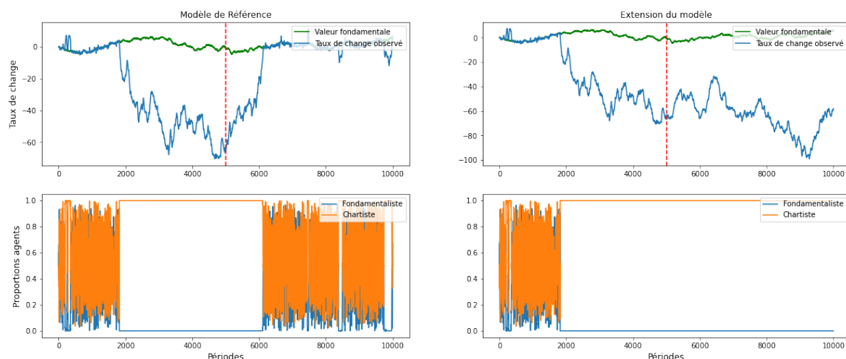
Figure 4.2.3 – Comparaison des dynamiques du taux de change et de la composition du marché pour l’extension (ajout des agents chartistes machine learner) et le modèle de référence - Exemple de période d’instabilité prolongée sans retour à l’équilibre suite à l’ajout des agents. La ligne verticale rouge correspond à la période durant laquelle la nouvelle heuristique est introduite.
