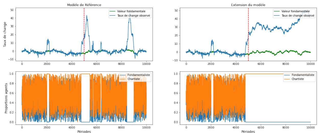
Figure 4.1.4 – Comparaison des dynamiques du taux de change et de la composition du marché pour l’extension (remplacement des agents chartistes) et le modèle de référence - Exemple de période d’instabilité prolongée suite au remplacement : pas de retour à l’équilibre - La ligne verticale rouge correspond à la période durant laquelle le remplacement des agents chartistes se produit.
