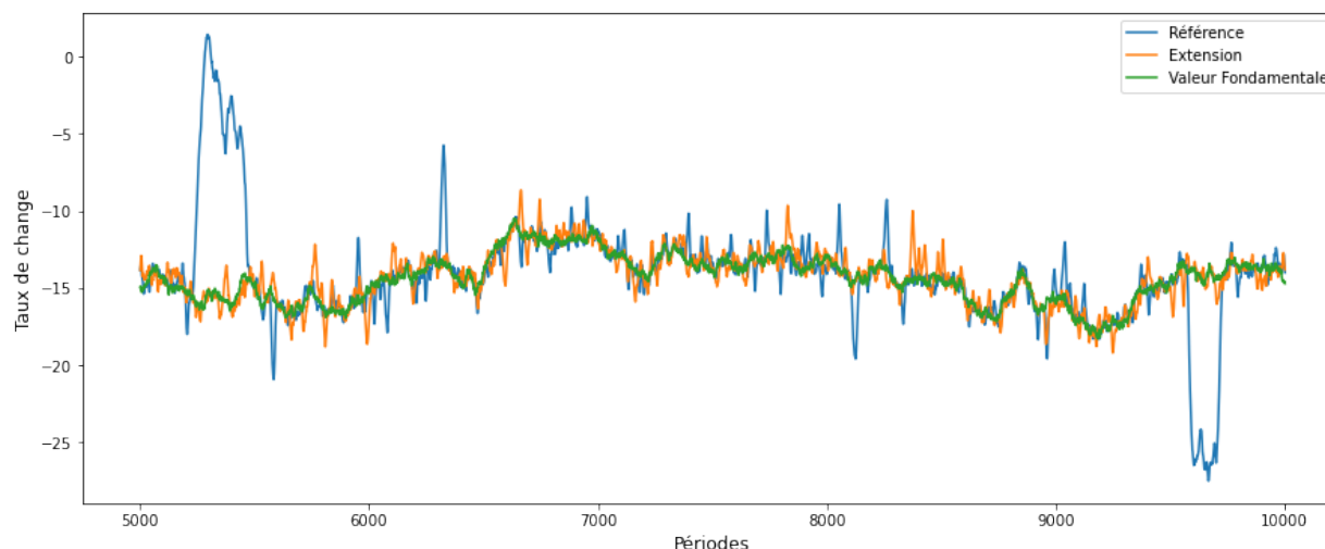
Figure 4.2.2 – Comparaison des dynamiques du taux de change générées par le modèle de référence et par l'extension (ajout des agents chartistes machine learner).
