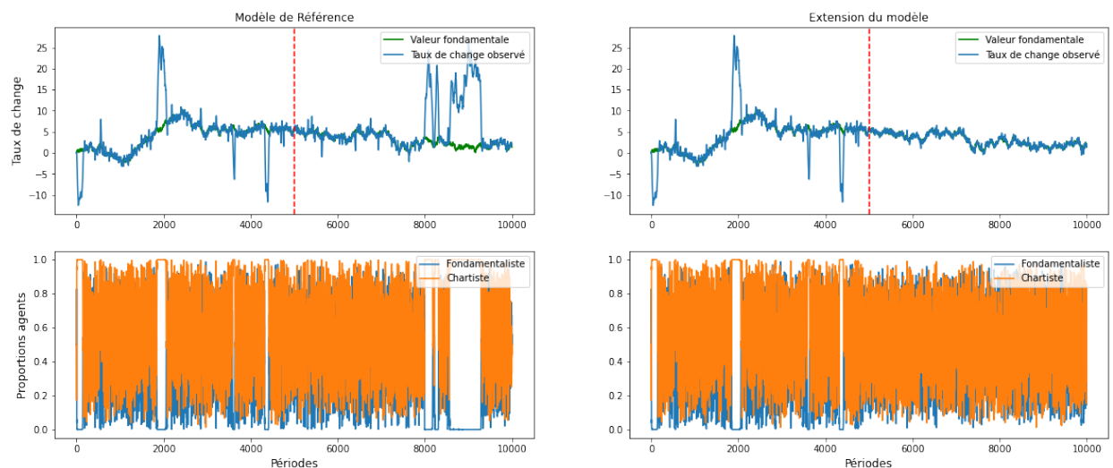
Figure 4.1.3 – Comparaison des dynamiques du taux de change et de la composition du marché pour l’extension (remplacement des agents chartistes) et le modèle de référence - Exemple de stabilité introduite par la nouvelle heuristique. La ligne verticale rouge correspond à la période durant laquelle le remplacement des agents chartistes se produit.
