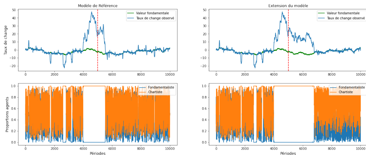
Figure 4.2.4 – Comparaison des dynamiques du taux de change et de la composition du marché pour l’extension (ajout des agents chartistes machine learner) et le modèle de référence - Exemple de période d’instabilité prolongée avec retour à l’équilibre suite à l’ajout des agents. La ligne verticale rouge correspond à la période durant laquelle la nouvelle heuristique est introduite.
