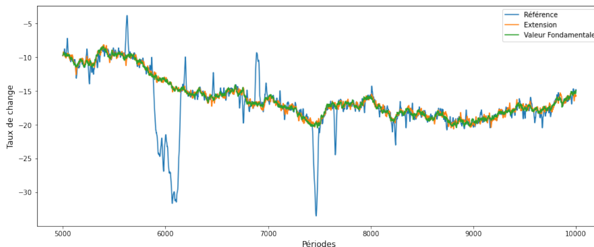
Figure 4.1.2 – Comparaison des dynamiques du taux de change générées par l'extension (remplacement des agents chartistes) et par le modèle de référence.
