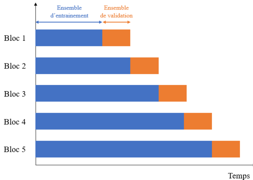
Figure 3.2.1 – Validation croisée à k blocs (« k -fold cross-validation ») pour séries temporelles. Dans notre modèle, k vaut 5 (généralement un k égal à 5 ou à 10 est utilisé).
