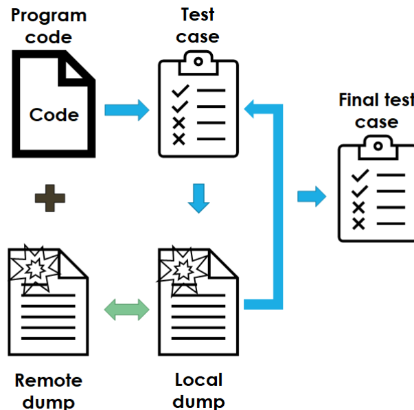
Figure 13: Fonctionnement de RECORE[39]
