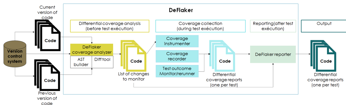
Figure 11: Fonctionnement de Deflaker[4]
