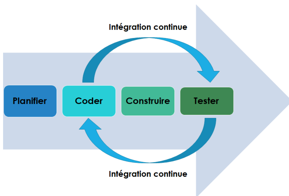
Figure 3: Schéma d'intégration continue[8]
