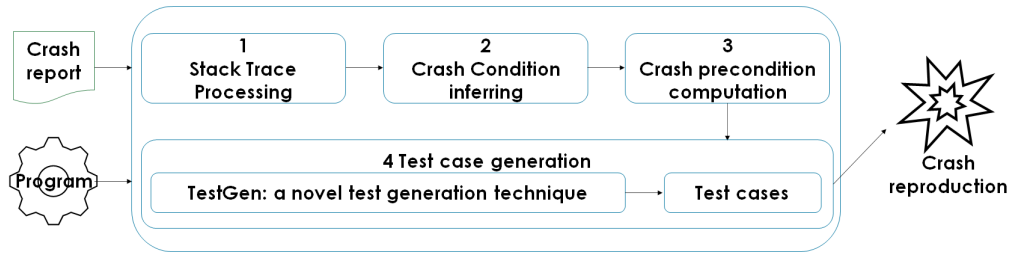
Figure 12: Architecture de STAR proposée par Chen & al.[7]
