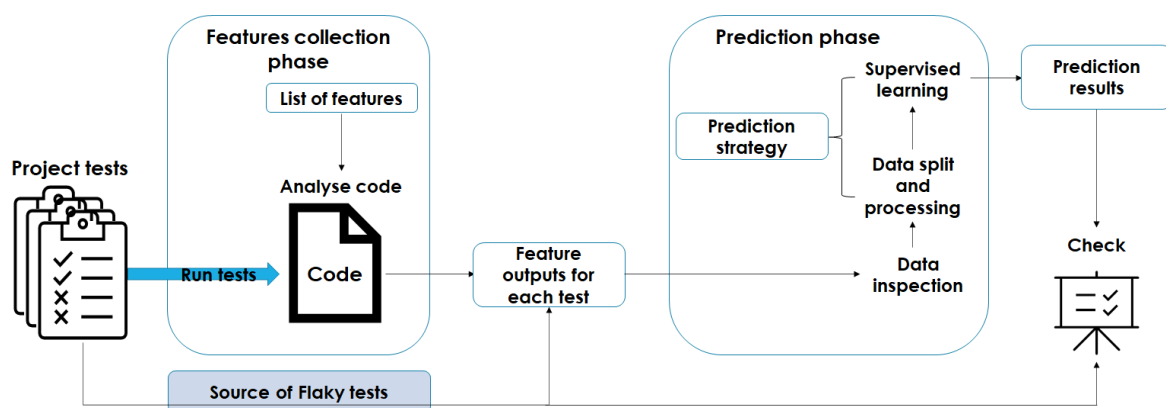
Figure 10: Fonctionnement de FlakeFlagger[2]
