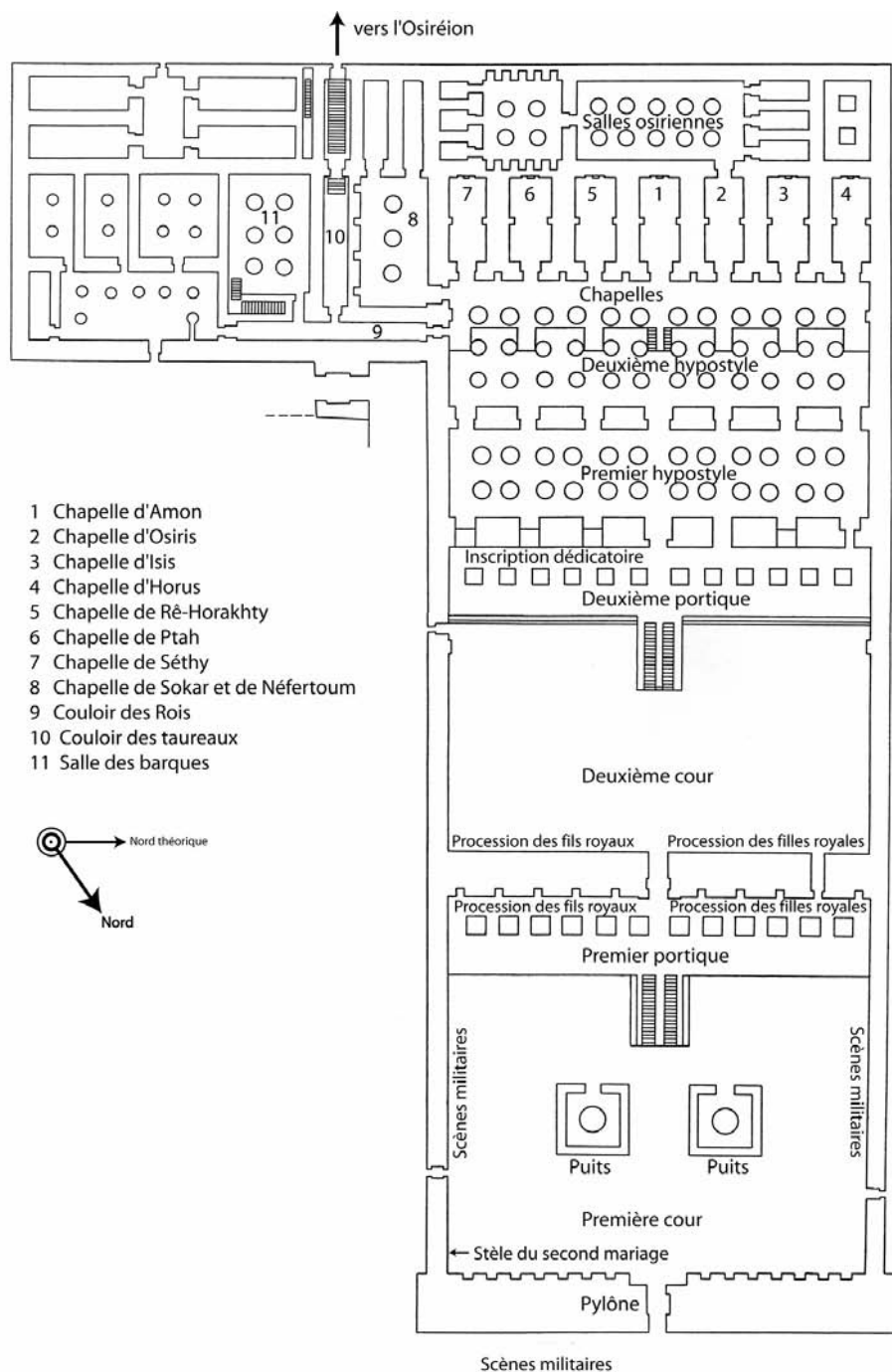
Fig. 9. Abydos. Plan du temple de Séthy I er (d'après PM VI, p. 2, 4, 22)
