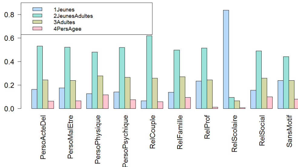
FIGURE 6.16 – Histogramme des âges en fonction du motif de la première consultation
