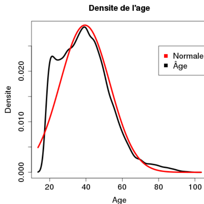
FIGURE 4.4 – Densité de l'âge et gaussienne associée
