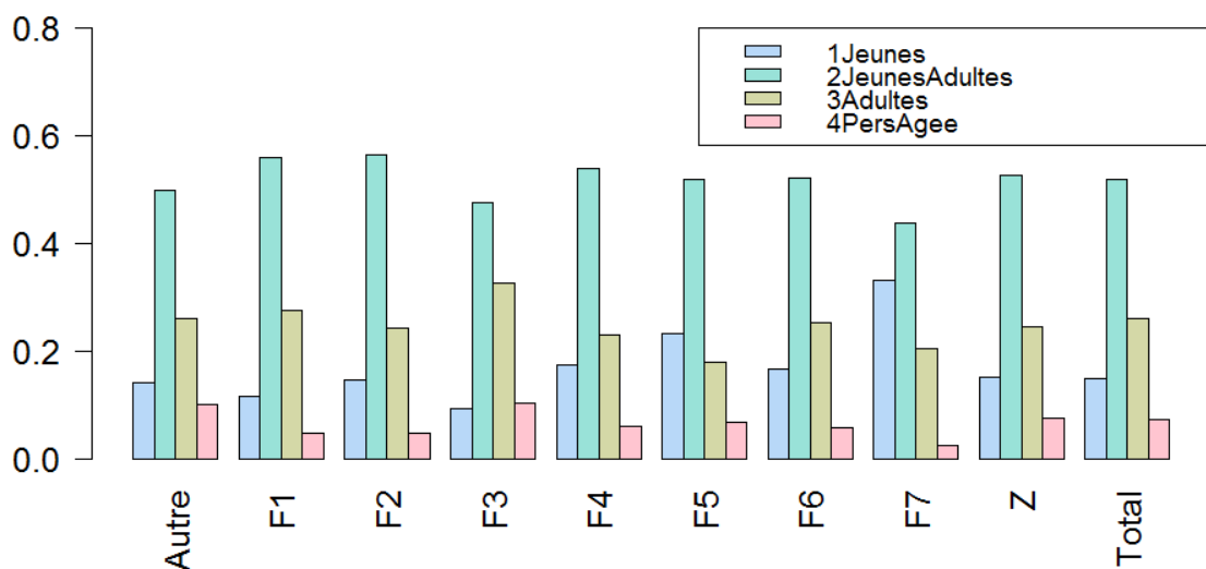
FIGURE 6.19 – Histogramme de l'âge en fonction du code
