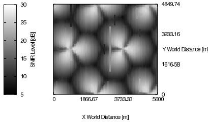
Fig. 9. SNIR map.
