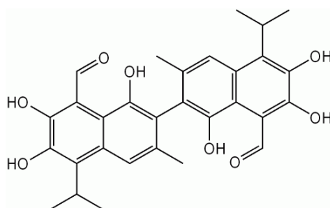
Fig. 7 : Formule chimique du gossypol ( C_{30}H_{30}O_8 ) : 2,2'-bis-(Formyl-1,6,7-trihydroxy-5-isopropyl-3-methylnaphthalene) ( www.en.wikipedia.org/wiki/Gossypol ).
