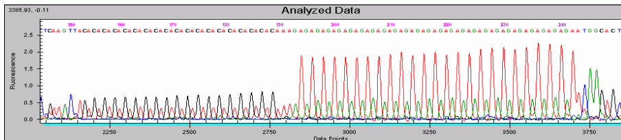
Figure 73 : Sortie microsatellite de séquenceur capillaire.
