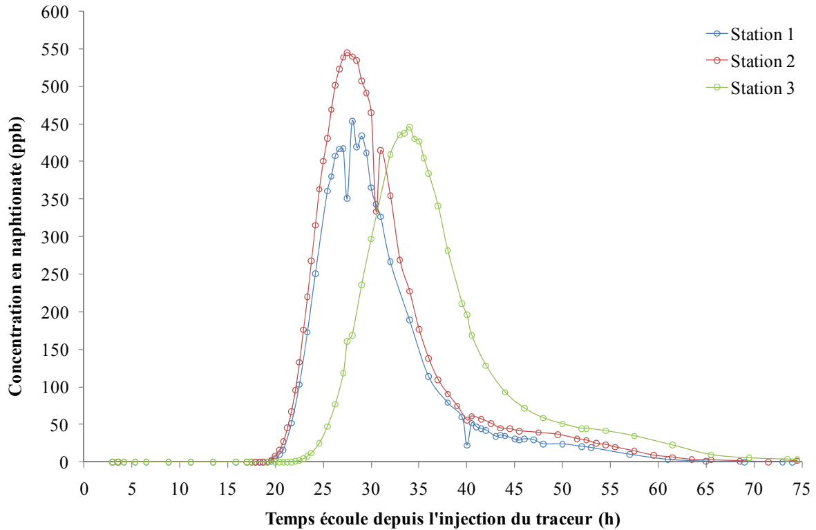
Fig.II.72 : Courbes de restitution du naphionate à la grotte –résurgence d'Herdal (stations 1 et 2) et aux résurgences du méandre recoupé (station 3).
