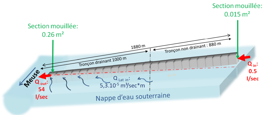
Fig.VII.15 : Modélisation Otis - Modèle conceptuel du système karstique "chantoir de Rostène – source de Bouvignes" – Q_{in} : Débit au site d'injection, Q_{out} : débit au site d'échantillonnage, Q_{Lat in} : Débit latéral entrant.
