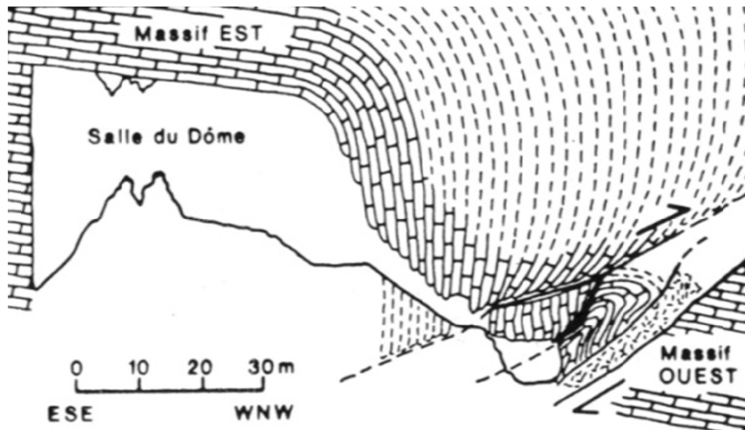
Fig.II.7 : Coupe schématique du pli-faille de la salle du Dôme (grotte de Han-sur-Lesse) décrit par Sorotchinsky (1939).
