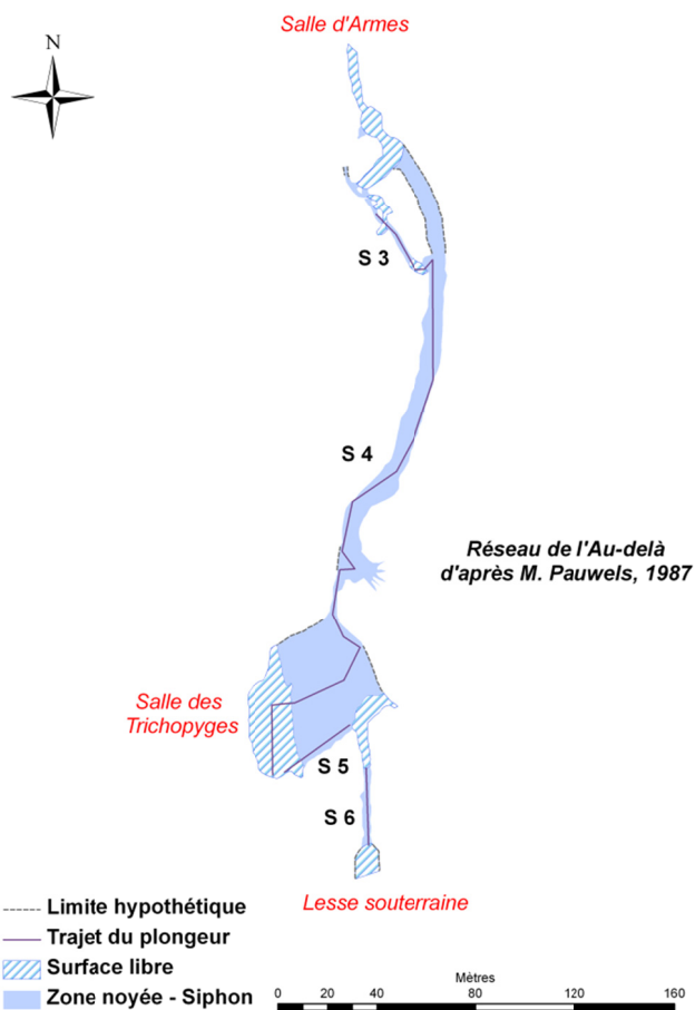
Fig. VI.13 : Topographie du réseau de l'Au-Delà – S3 à S6: dénomination des zones noyée (Pauwels, 1987).
