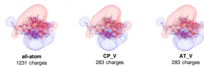
Fig. 5 MEP isocontours of Ubiquitin: -0.05, +0.05 e/bohr.
