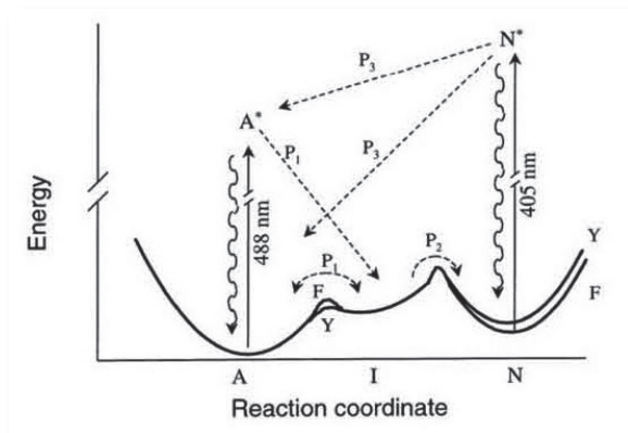
Fig. 3 11 : GFP dans l'état A est excitée vers l'état A* et retourne à l'état A en émettant un photon. Quand on atteint le point I à partir de A, il n'y a plus de fluorescence à moins que la molécule passe de l'état I à l'état A. Quand la molécule passe de l'état I à l'état N, il n'y a pas non plus de fluorescence à moins que la molécule passe de l'état N à l'état N* par absorption d'un rayonnement à 405 nm et la GFP retourne à l'état A ou A*.
