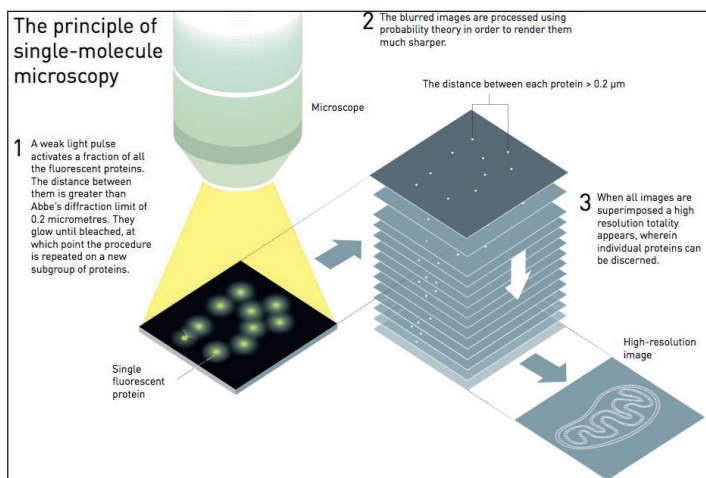
Fig. 4 : Le principe du microscope «mono-moléculaire» 16 .
