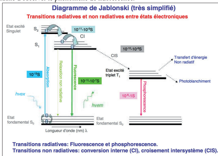
Fig. 1 : Diagramme de Jablonski 4
