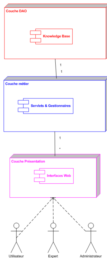
FIG. 5.3 – Diagramme de déploiement de S3^m DSS
