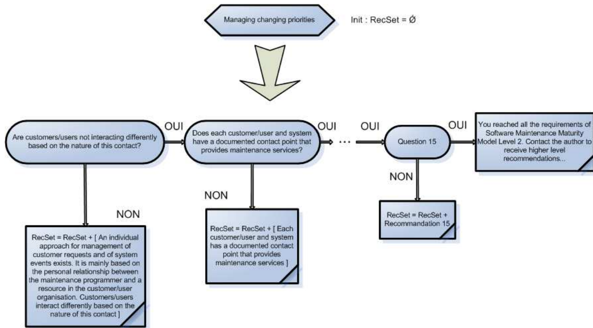
FIG. 2.7 – Exemple 2 : Arbre de décision orienté déduction
