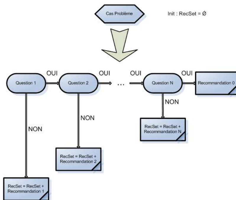
FIG. 2.2 – Arbre de décision orienté déduction
