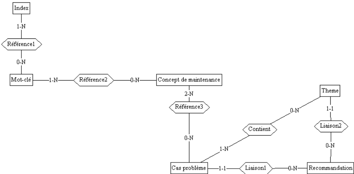
FIG. 4.11 – Schéma conceptuel de S3^m DSS
