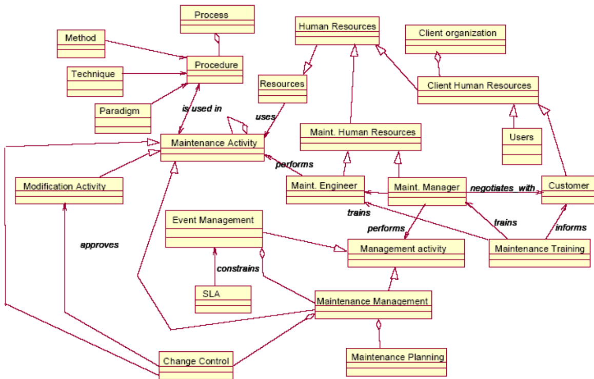
FIG. 2.4 – Partie de l'ontologie de la maintenance du logiciel, tiré de [14]
