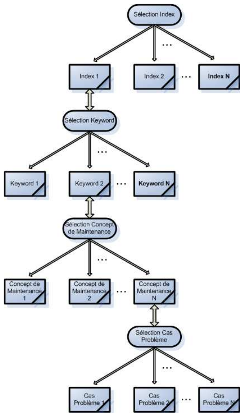
FIG. 2.1 – Arbre de décision orienté sélection
