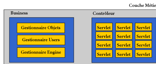
FIG. 5.5 – Structure de la couche Business de S3^m DSS
