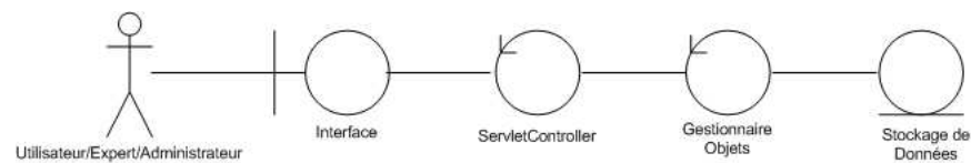
FIG. 4.2 – Diagramme de robustesse - Consultation KB
