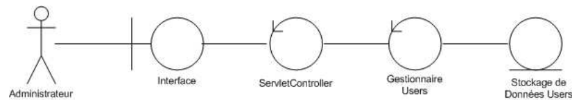
FIG. 4.3 – Diagramme de robustesse - Ajout compte
