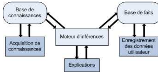
FIG. 2.6 – Représentation d'un système expert, adapté de [10]
