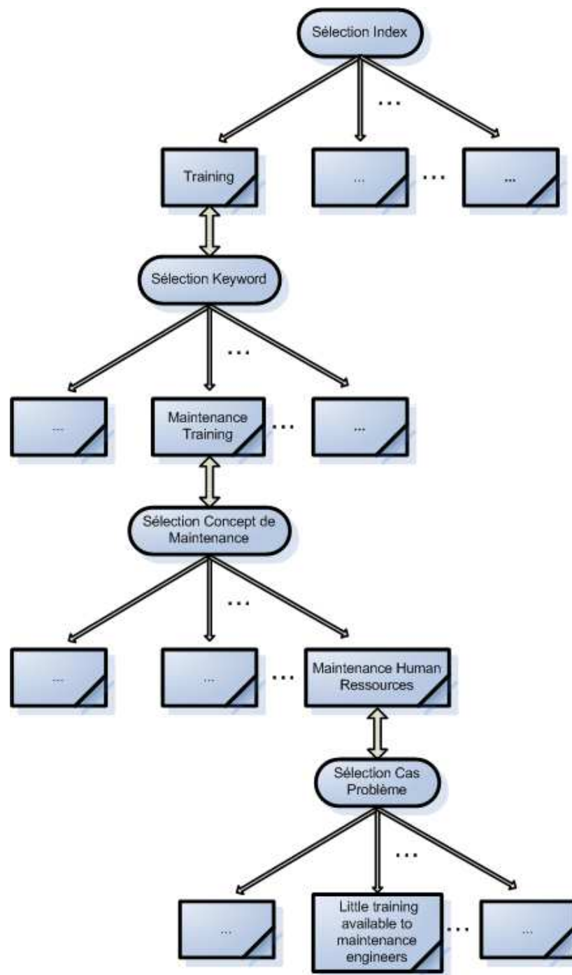
FIG. 2.4 – Exemple 1 : Arbre de décision orienté sélection
