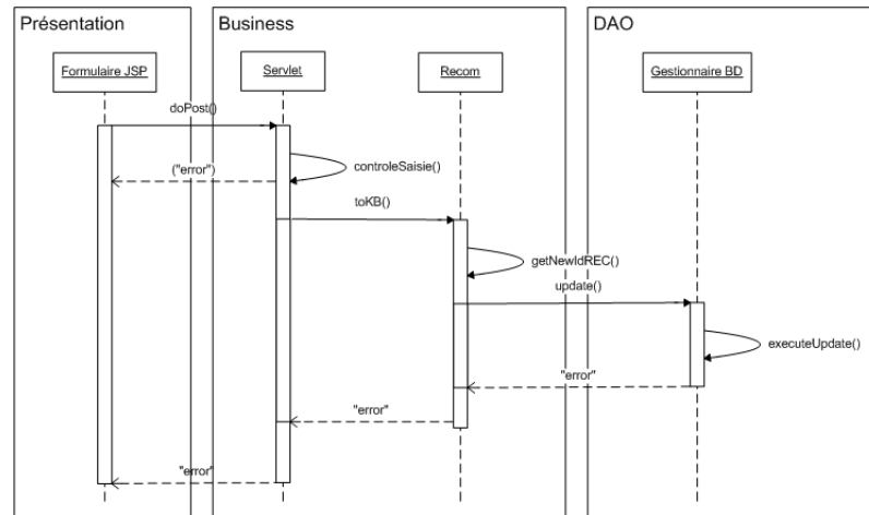
FIG. 4.9 – Diagramme de séquence - Ajout KB
