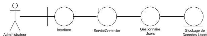
FIG. 8 – Diagramme de robustesse - Retrait compte
