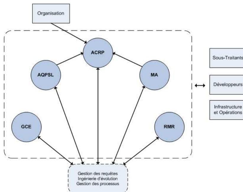
FIG. 2.15 – Interactions des KPAs du support à l'ingénierie d'évolution, adapté de [3]
