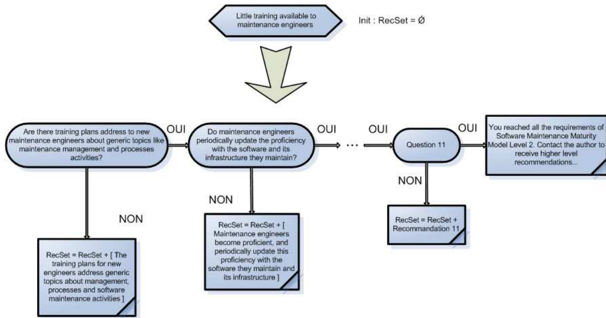
FIG. 2.5 – Exemple 1 : Arbre de décision orienté déduction
