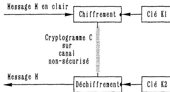
Figure 6 : Schéma de chiffrement asymétrique.
