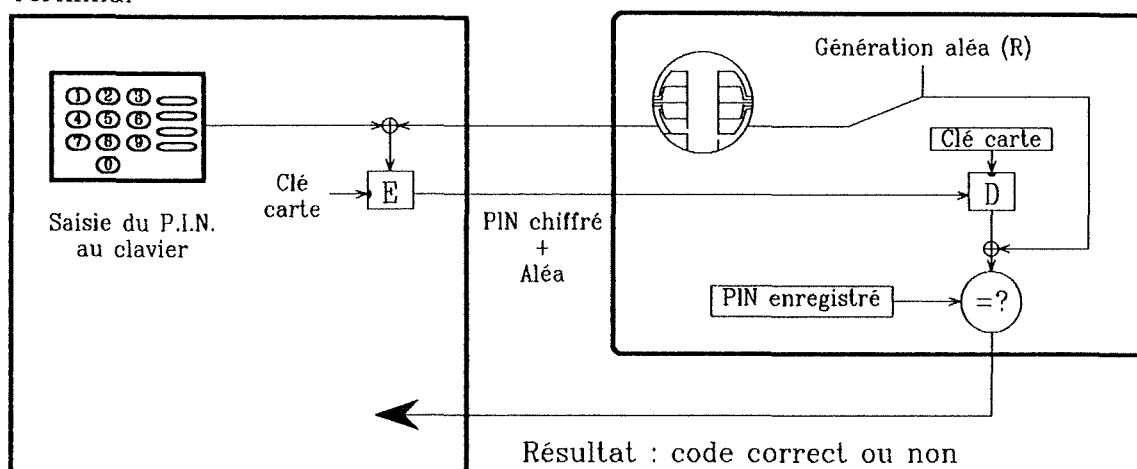
Figure 23 : Identification avec algorithme de chiffrement.
