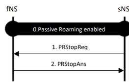
FIGURE 2.7 – Fin de Roaming
