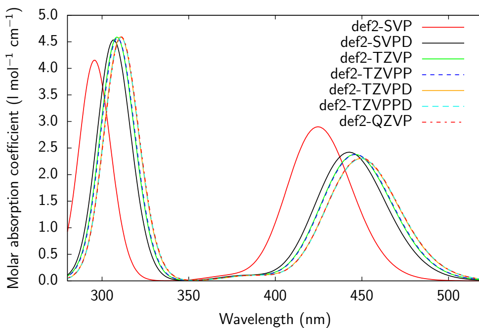
(b) Keto
