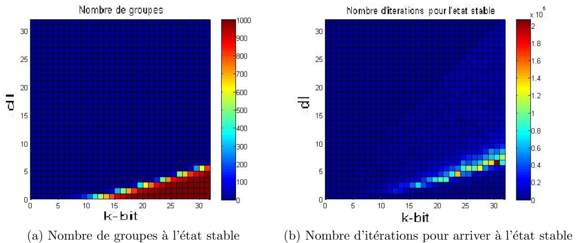
FIGURE 2.5 – La figure de gauche représente le nombre de groupes qui sont formés à la fin de l'algorithme et la figure de droite désigne le nombre d'itérations nécessaires à la réalisation de cette algorithme.
