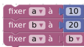
FIGURE 7.7 – Duplicata de la question 1 de Dehnadi traduite en langage de programmation par blocs
